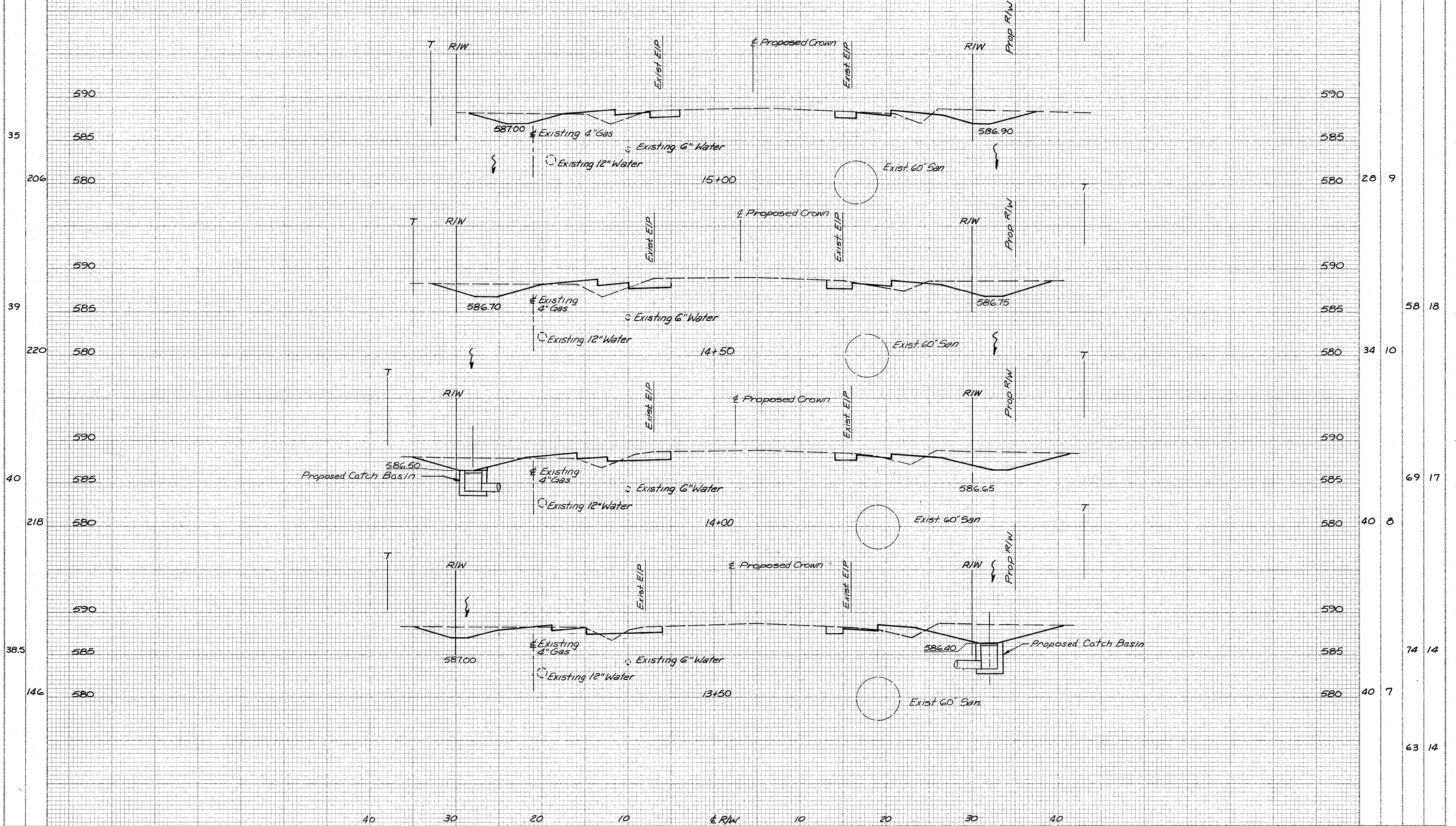
ERIE RD. X-SECTIONS - STA 13+50 TO STA 15+00
