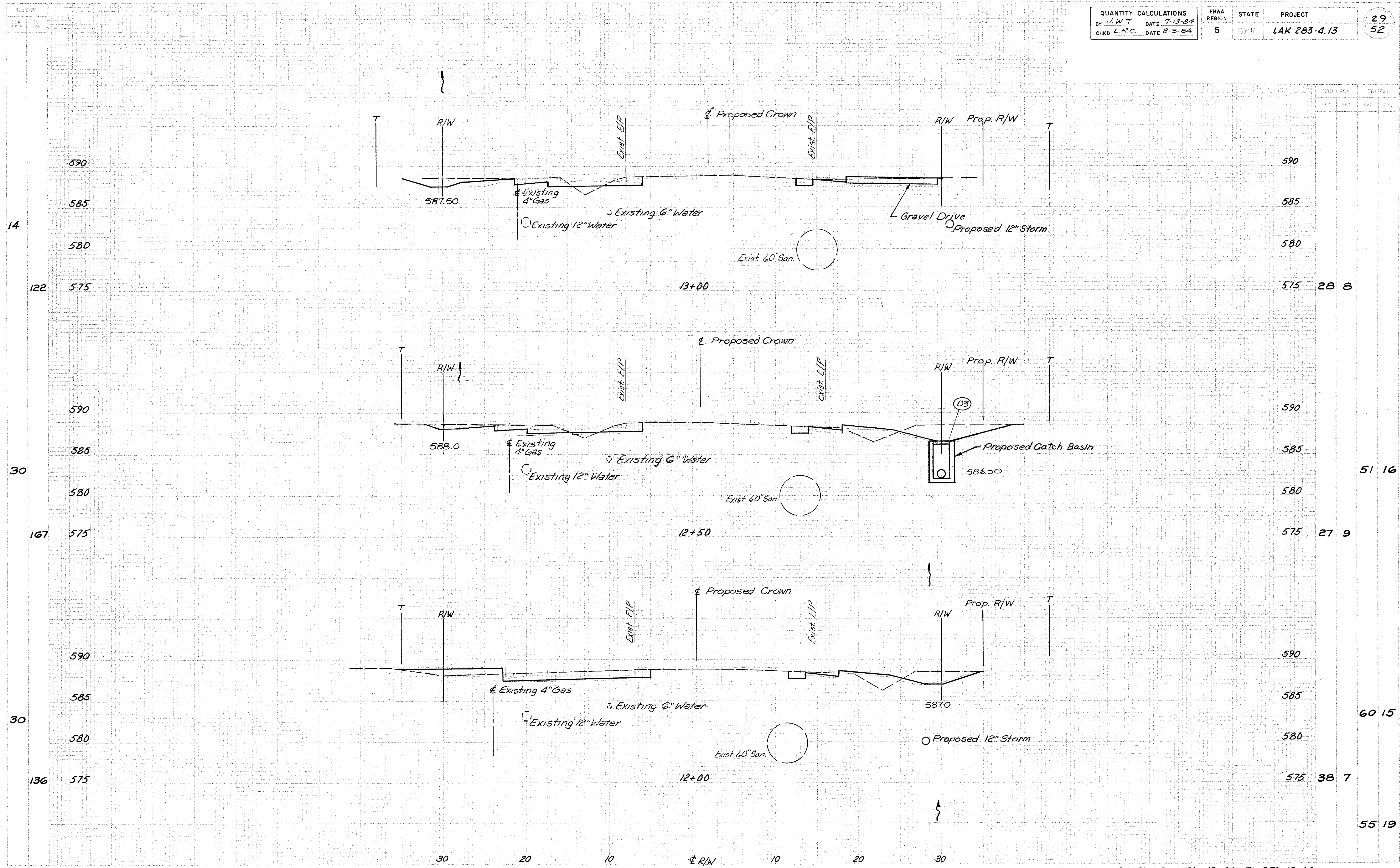
ERIE RD. X-SECTIONS - STA. 12+00 TO STA. 13+00
