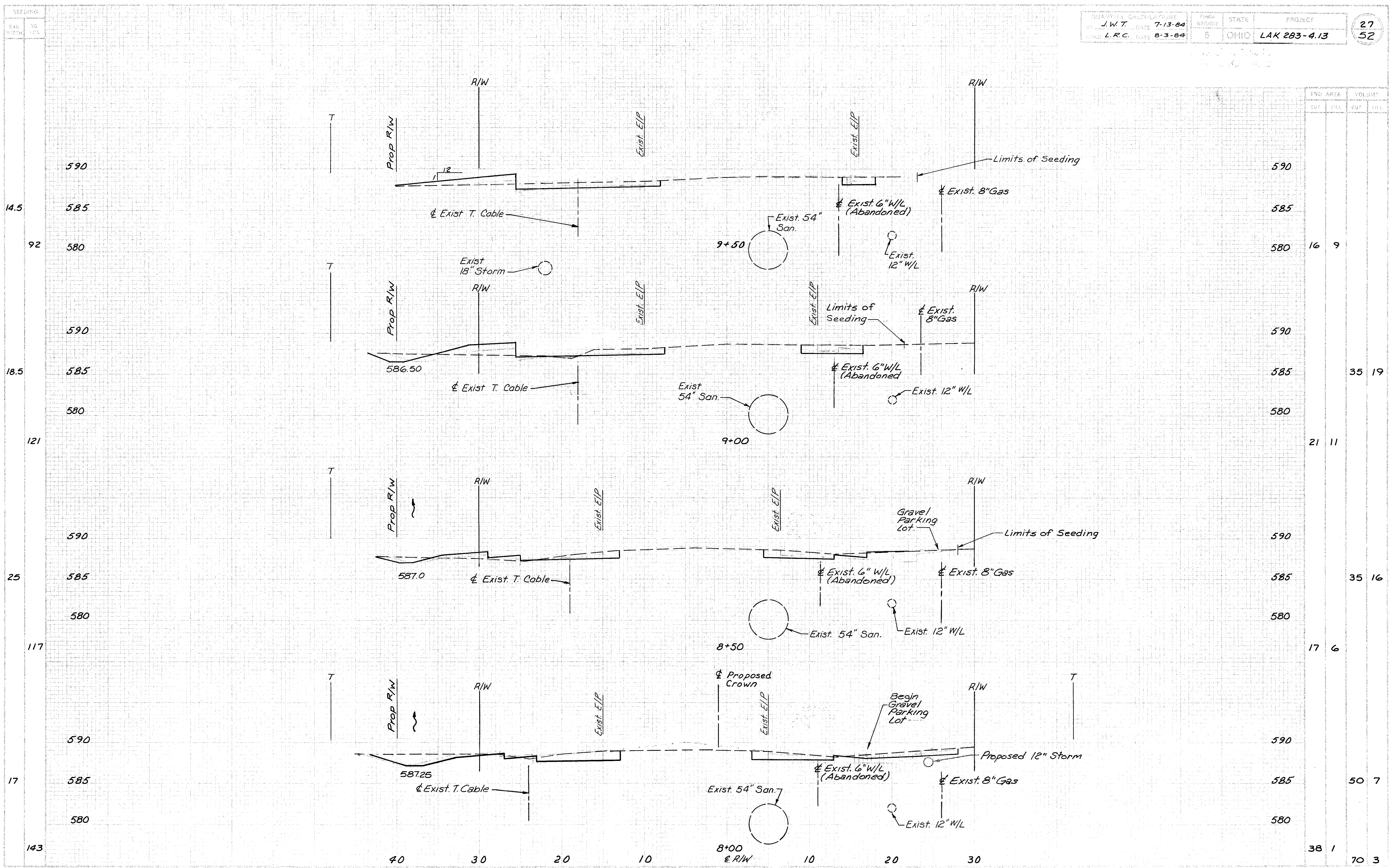
ERIE RD. X-SECTIONS - STA. 8+00 TO STA. 9+50
