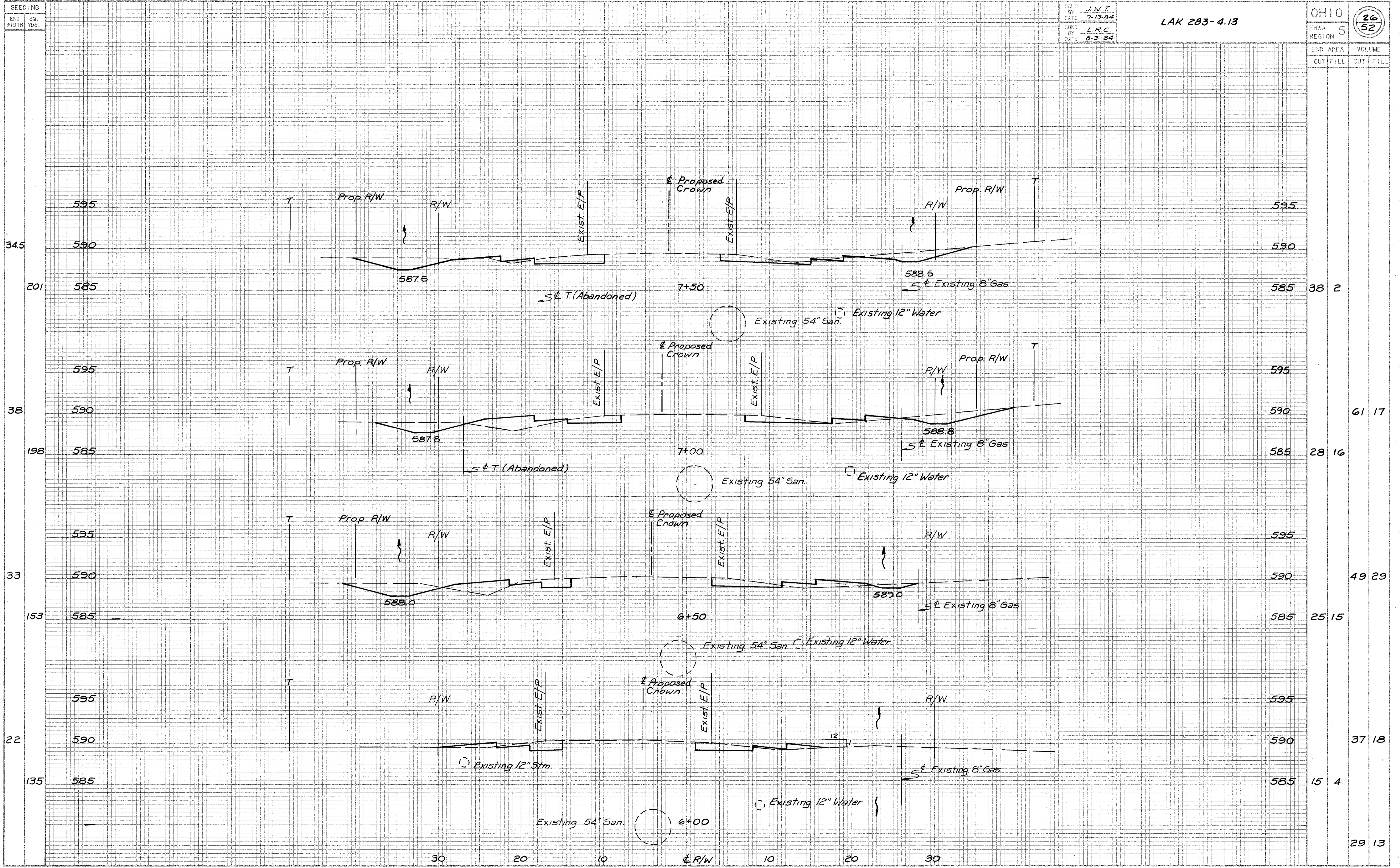
ERIE RD. X-SECTIONS - STA. 6+00 TO STA. 7+50
