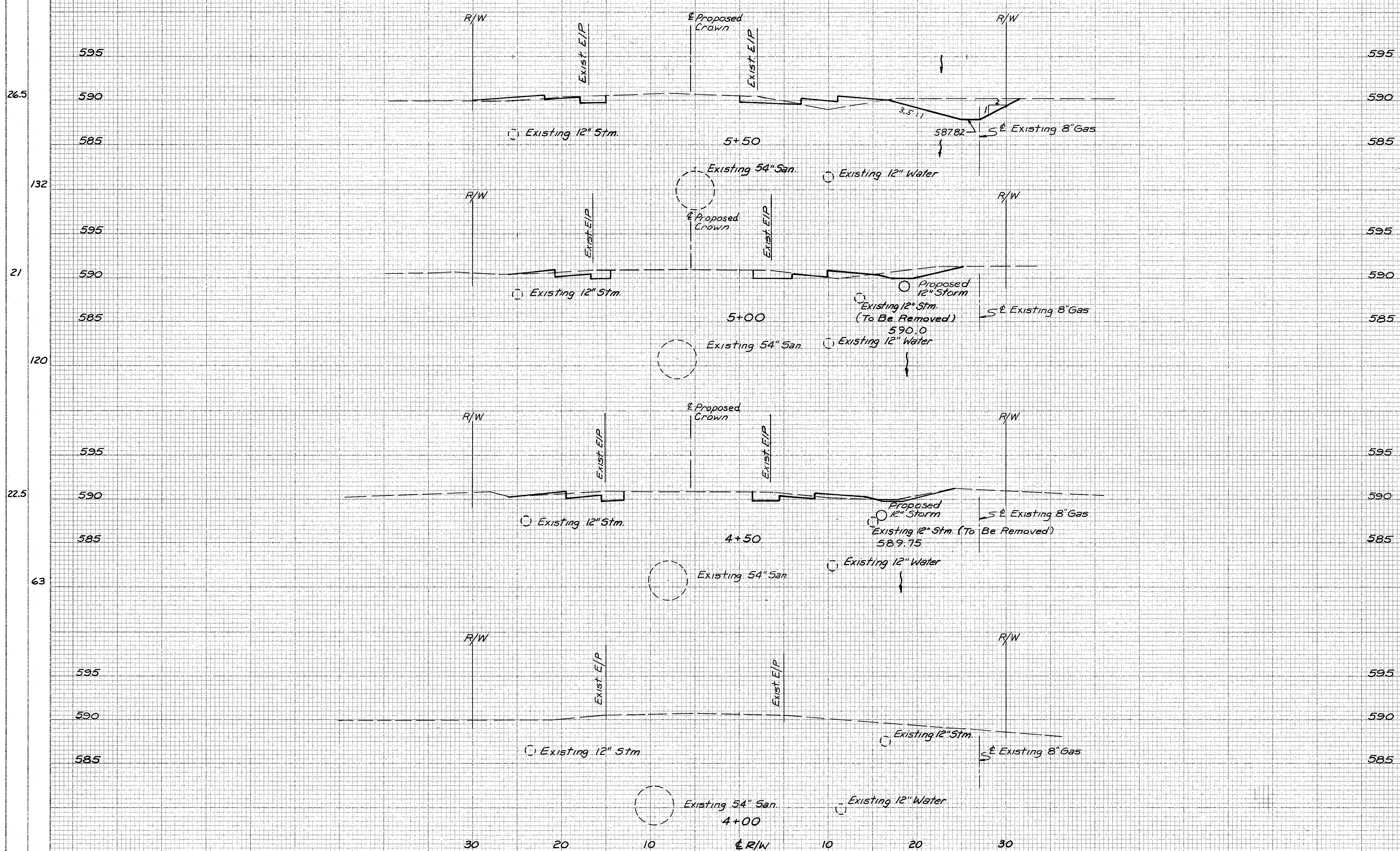
ERIE RD X-SECTIONS - STA. 4+00 TO STA. 5+50
