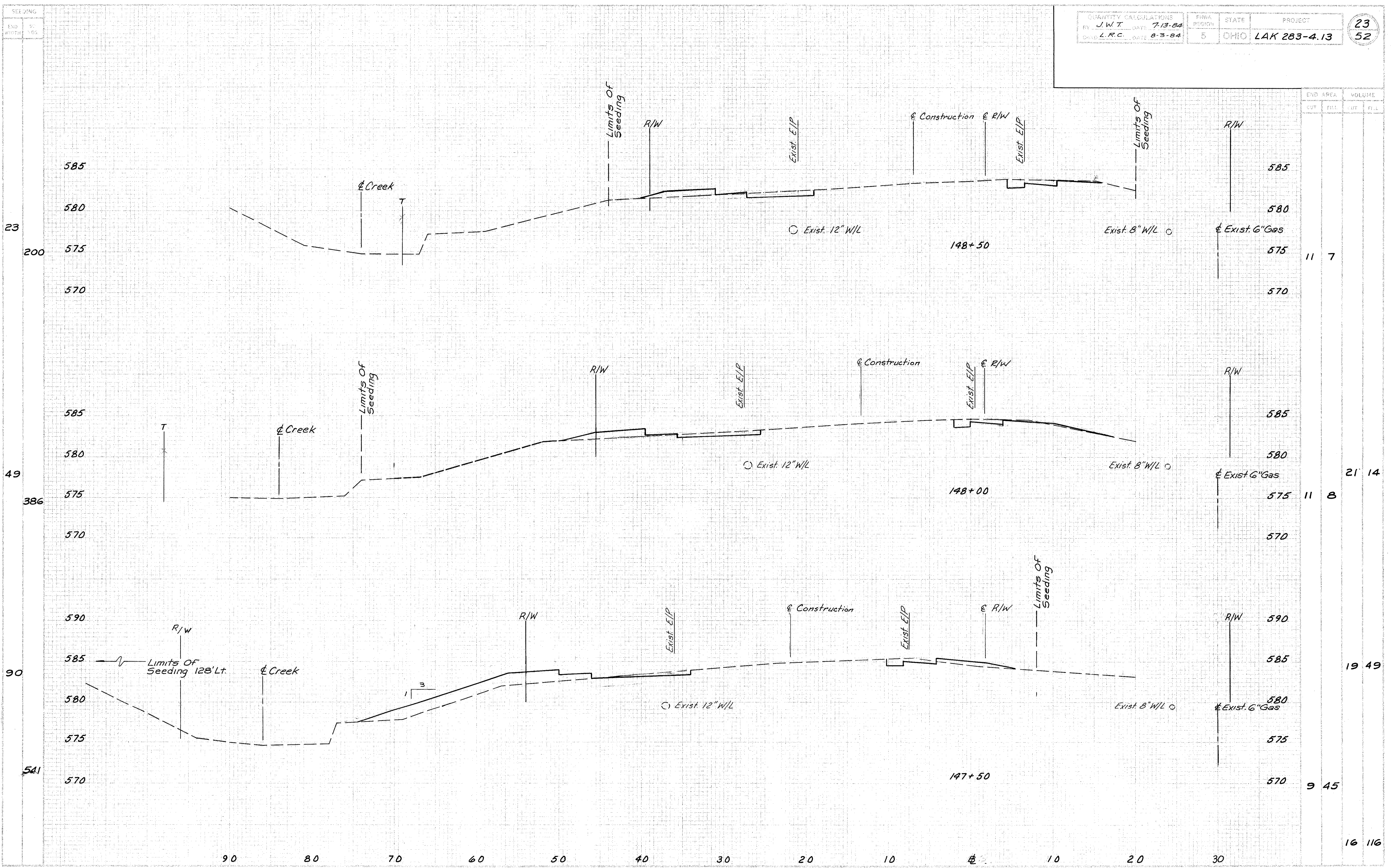
SR. 283 X-SECTIONS- STA 147+50 TO STA 148+50
