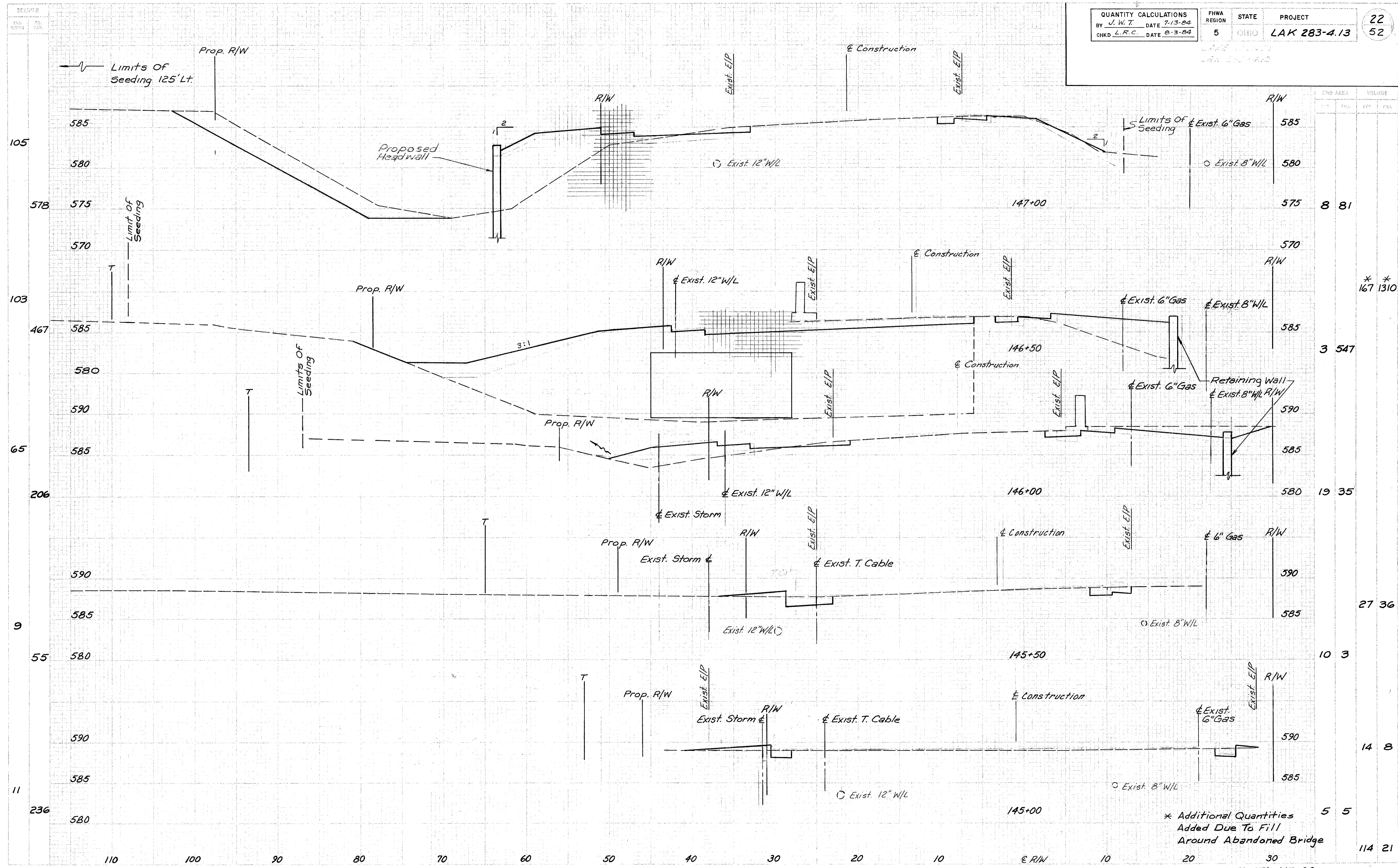
SR. 283 X-SECTIONS - STA. 145+00 TO STA. 147+00
