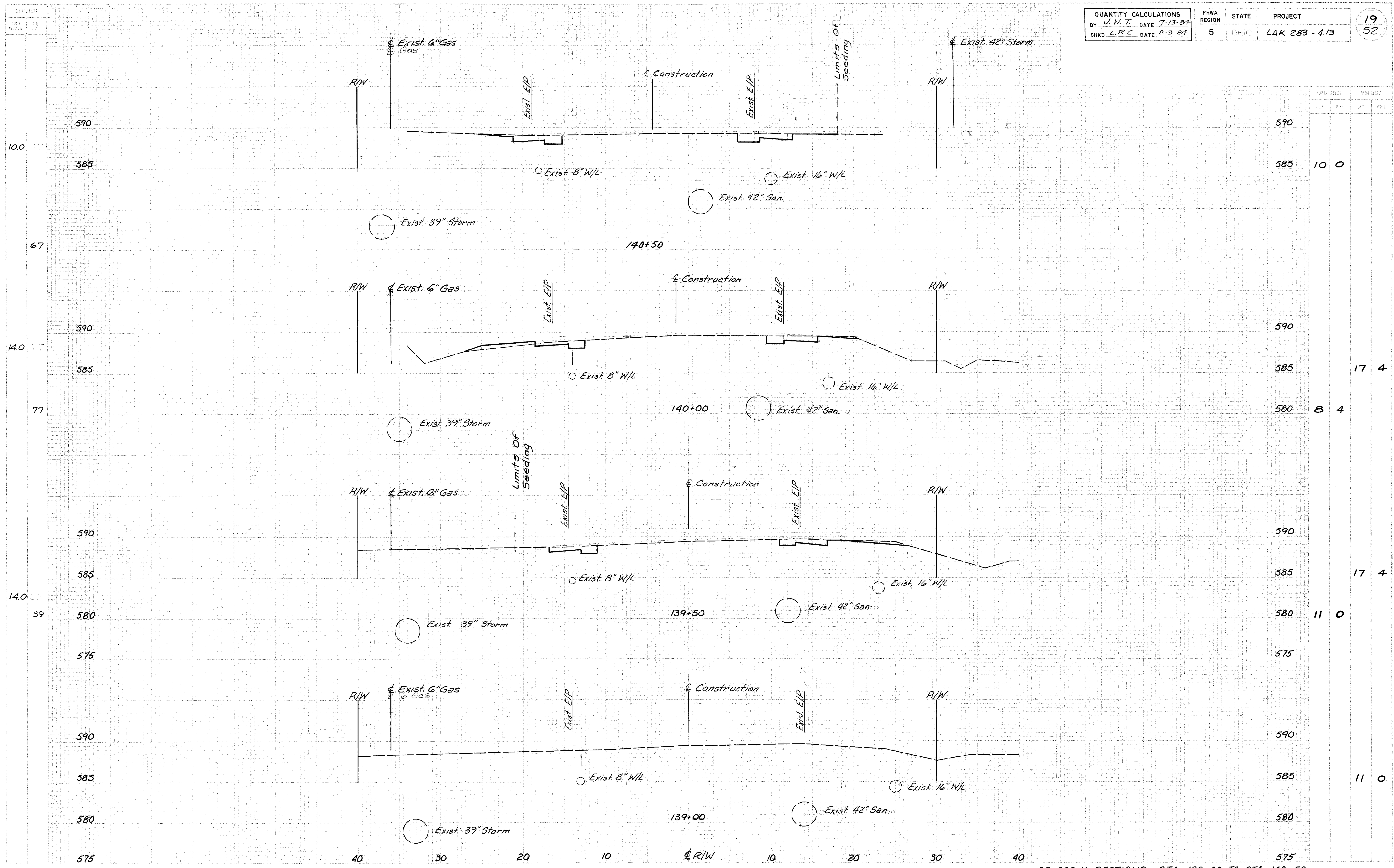
SR. 283 X-SECTIONS - STA. 139+00 TO STA. 140+50
