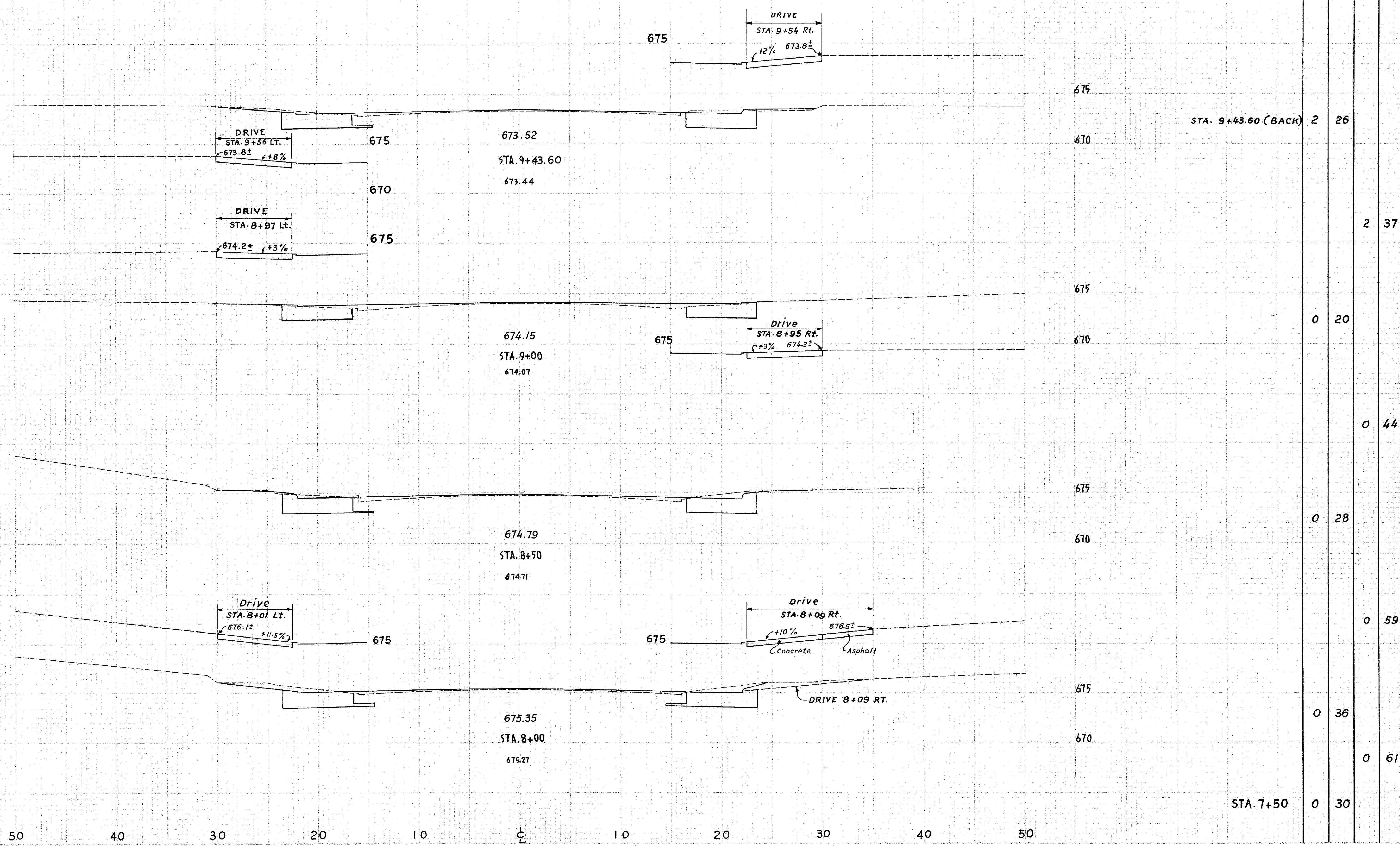
CROSS SECTIONS ... STA. 8+00 to STA. 9+43.60
