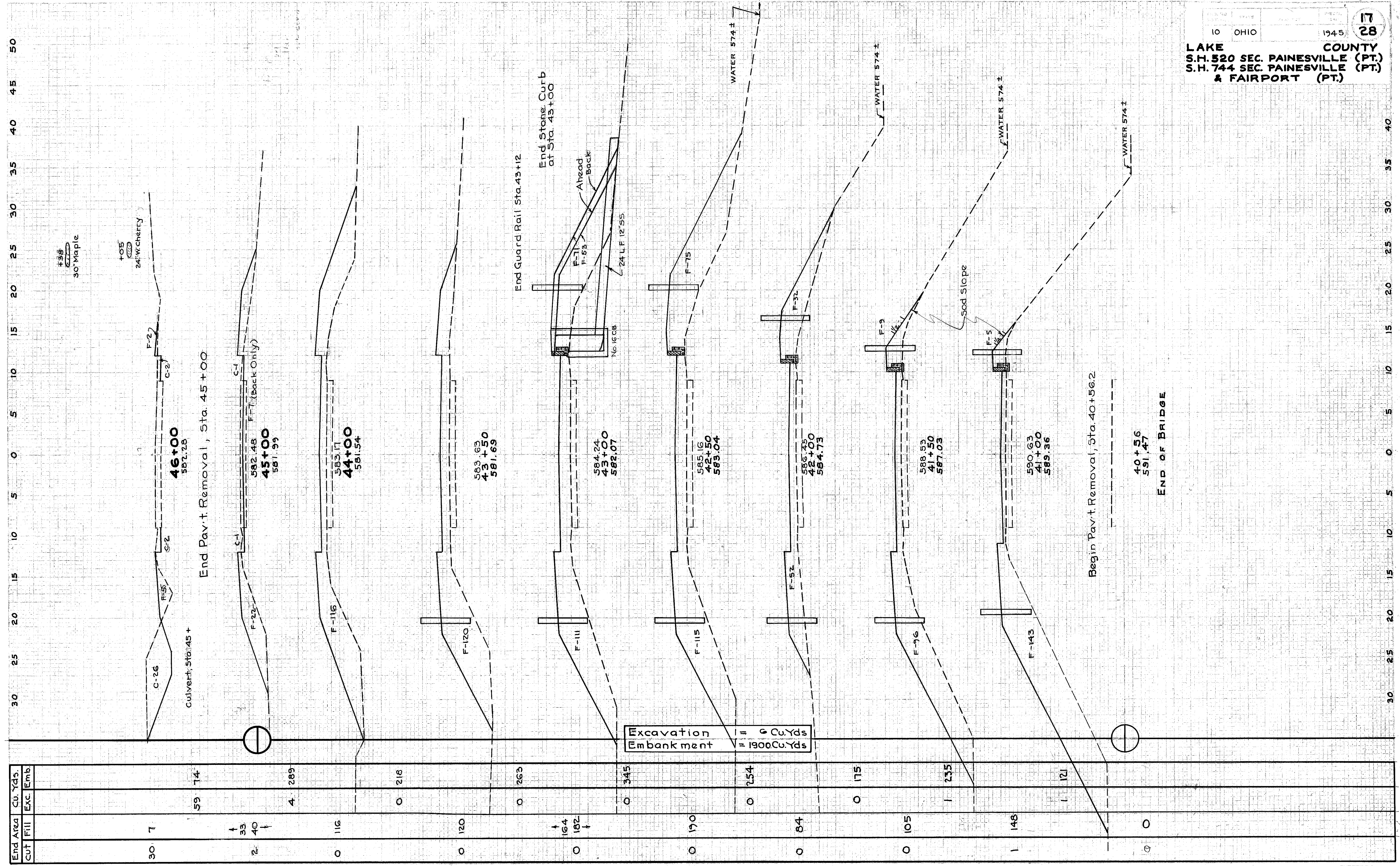
CROSS SECTIONS STA. 40+56 TO STA. 46+00
