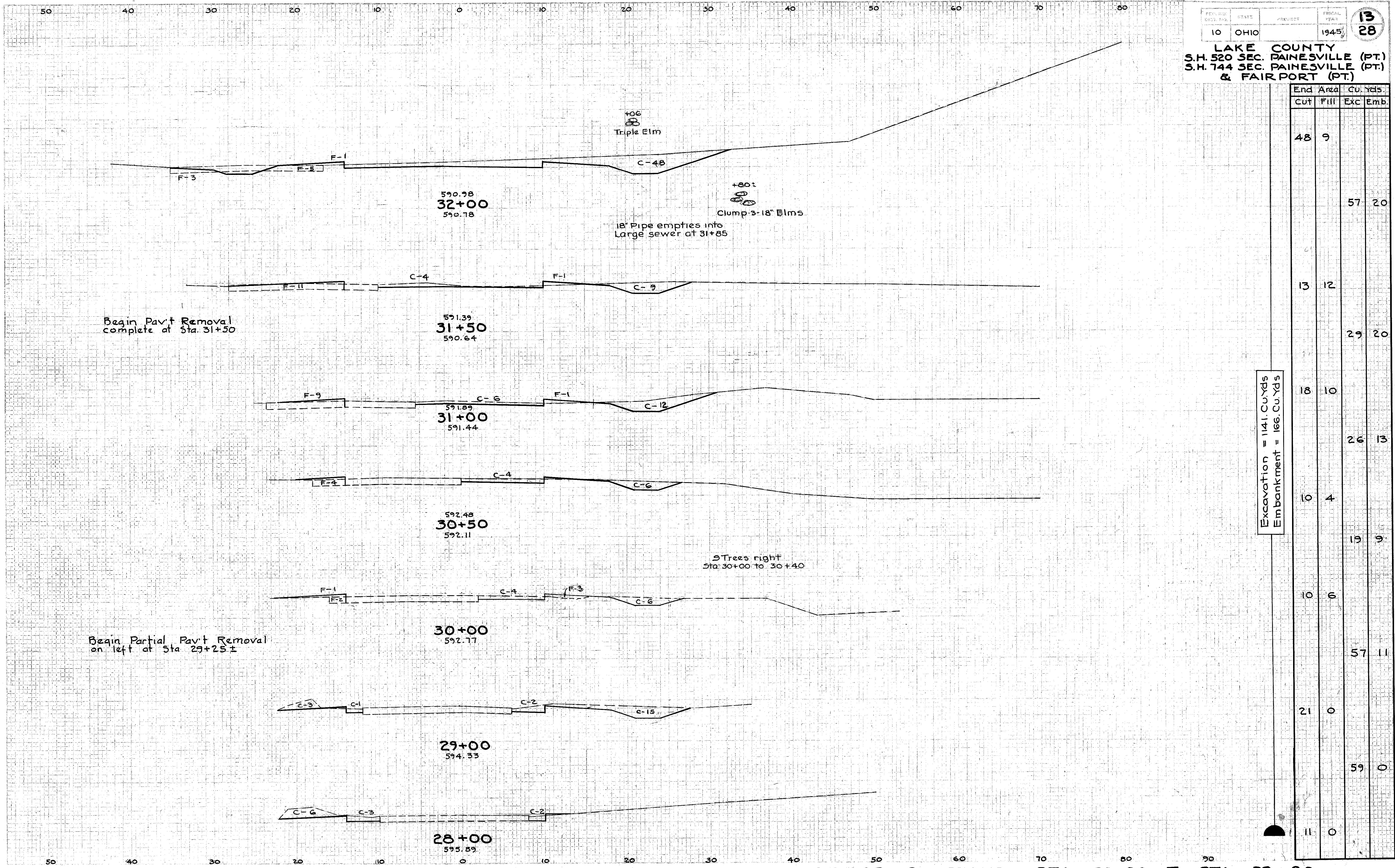
CROSS SECTIONS STA. 28+00 To STA. 32+00
