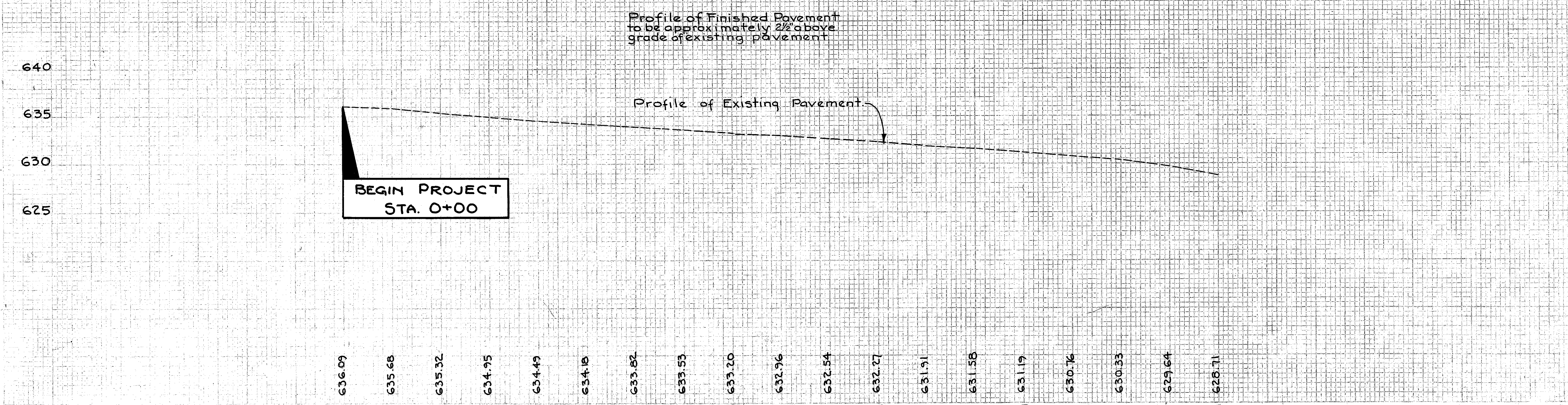
PLAN & PROFILE STA. 0+00 TO STA. 9+00
