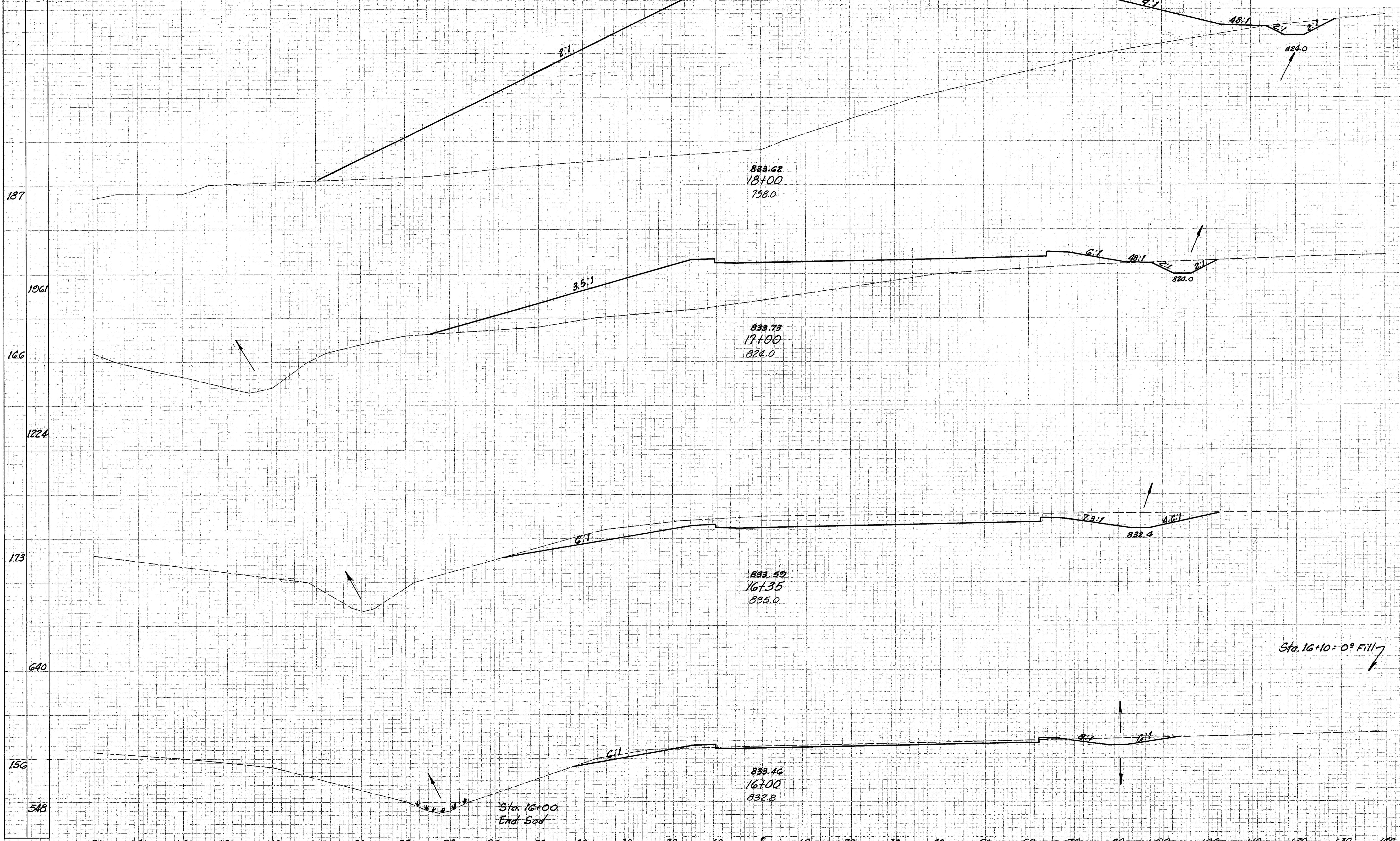
EUCLID SPUR INTERCHANGE - Ramp "D" Sta. 16+00 To Sta. 18+00
