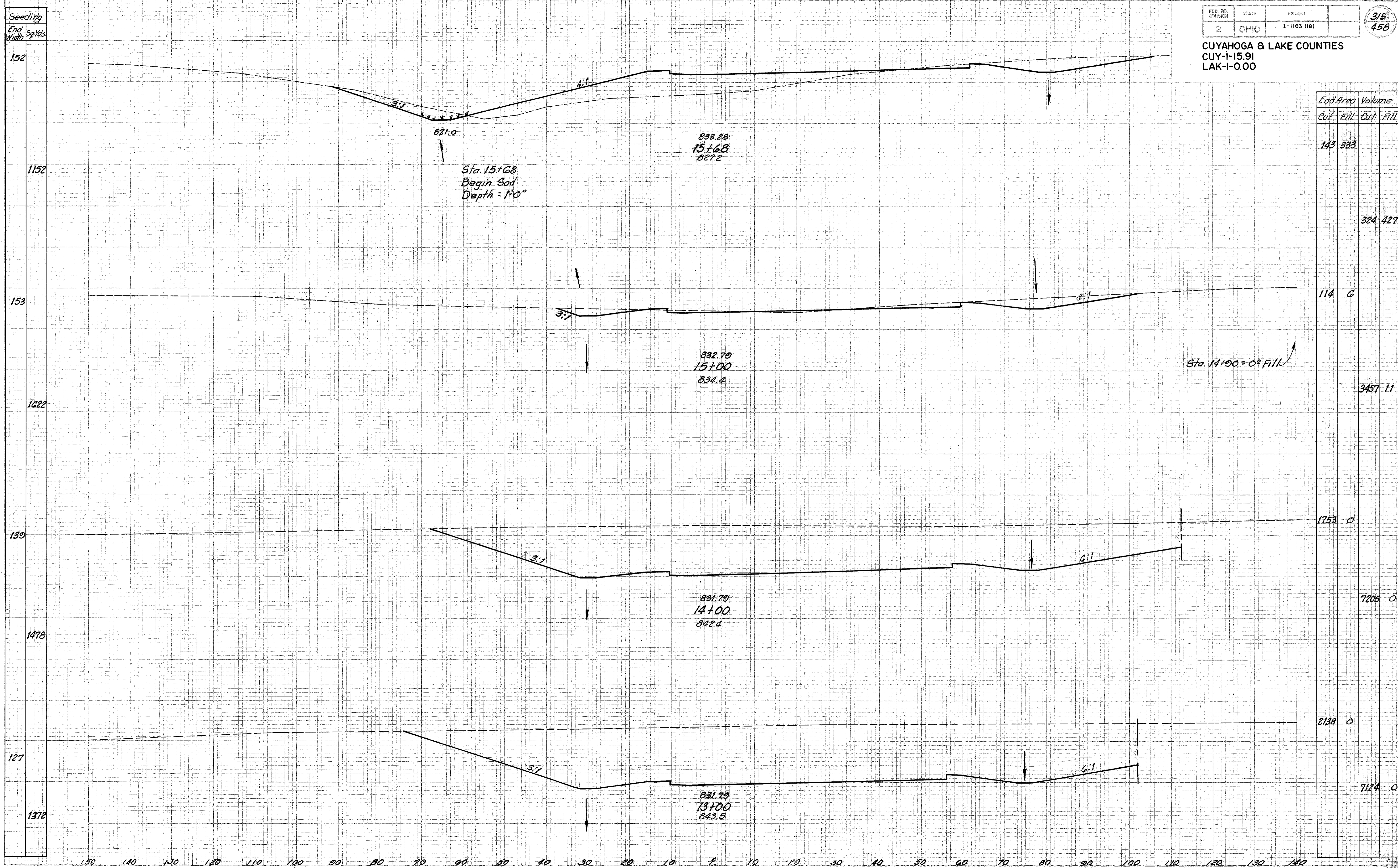
EUCLID SPUR INTERCHANGE - Ramp "D" Sta. 13+00 To Sta. 15+68
