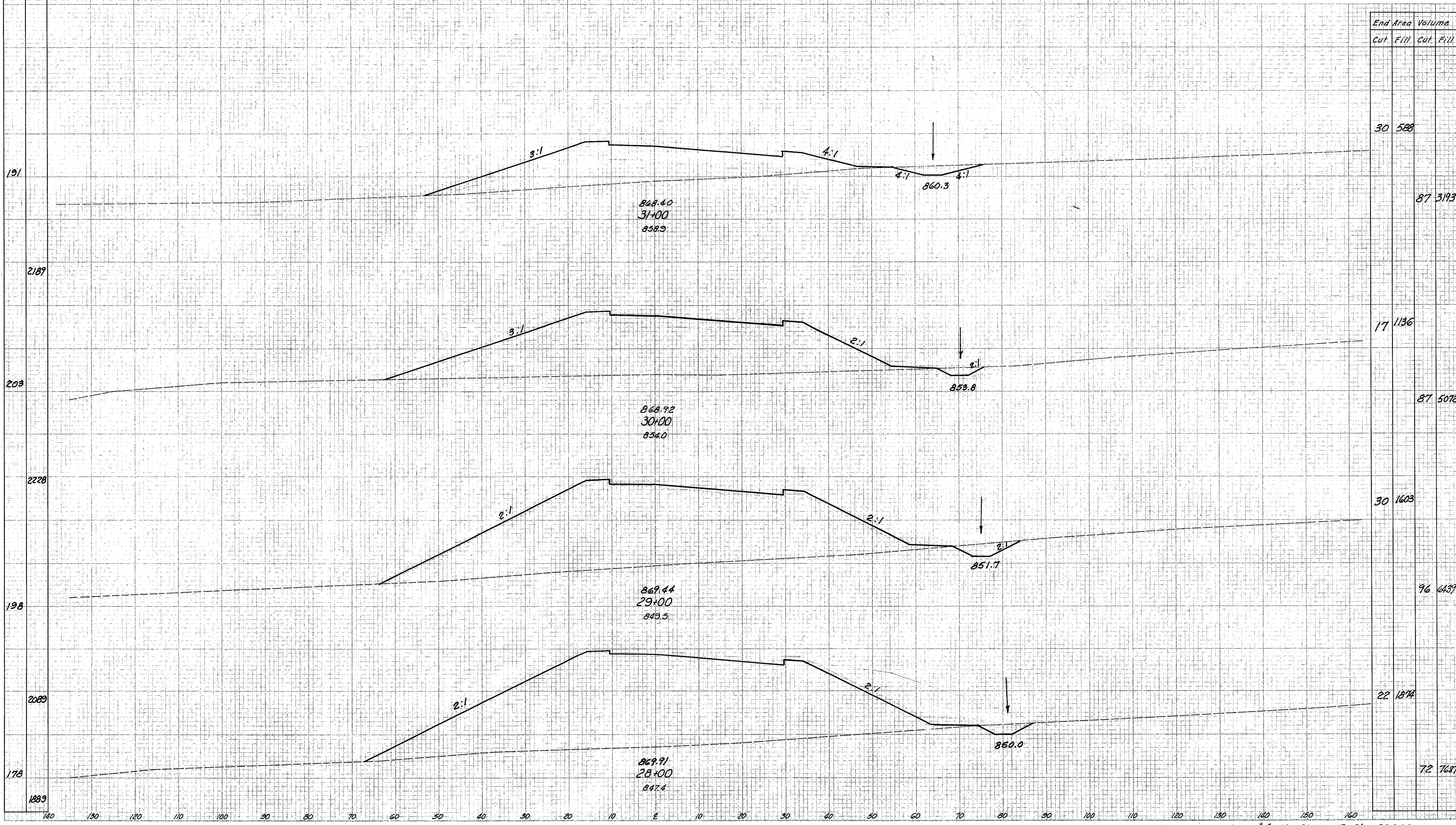
EUCLID SPUR INTERCHANGE - Ramp "C" Sta. 28+00 To Sta. 31+00
