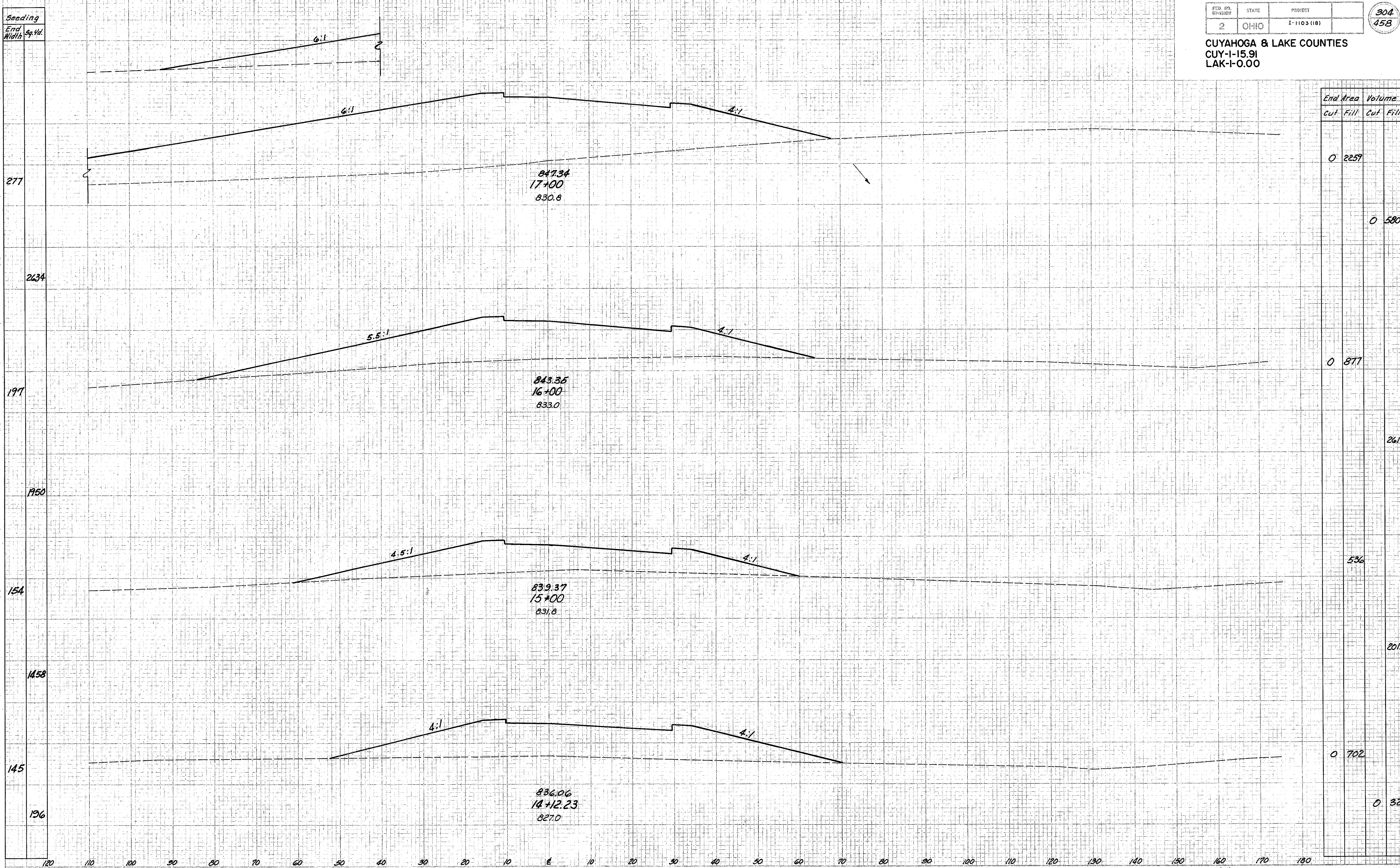
EUCLID SPUR INTERCHANGE - Ramp "C" Sta. 14+12.23 To Sta. 17+00
