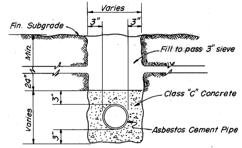
ONE WAY DUCT SECTION Scale: 1" = 1'
