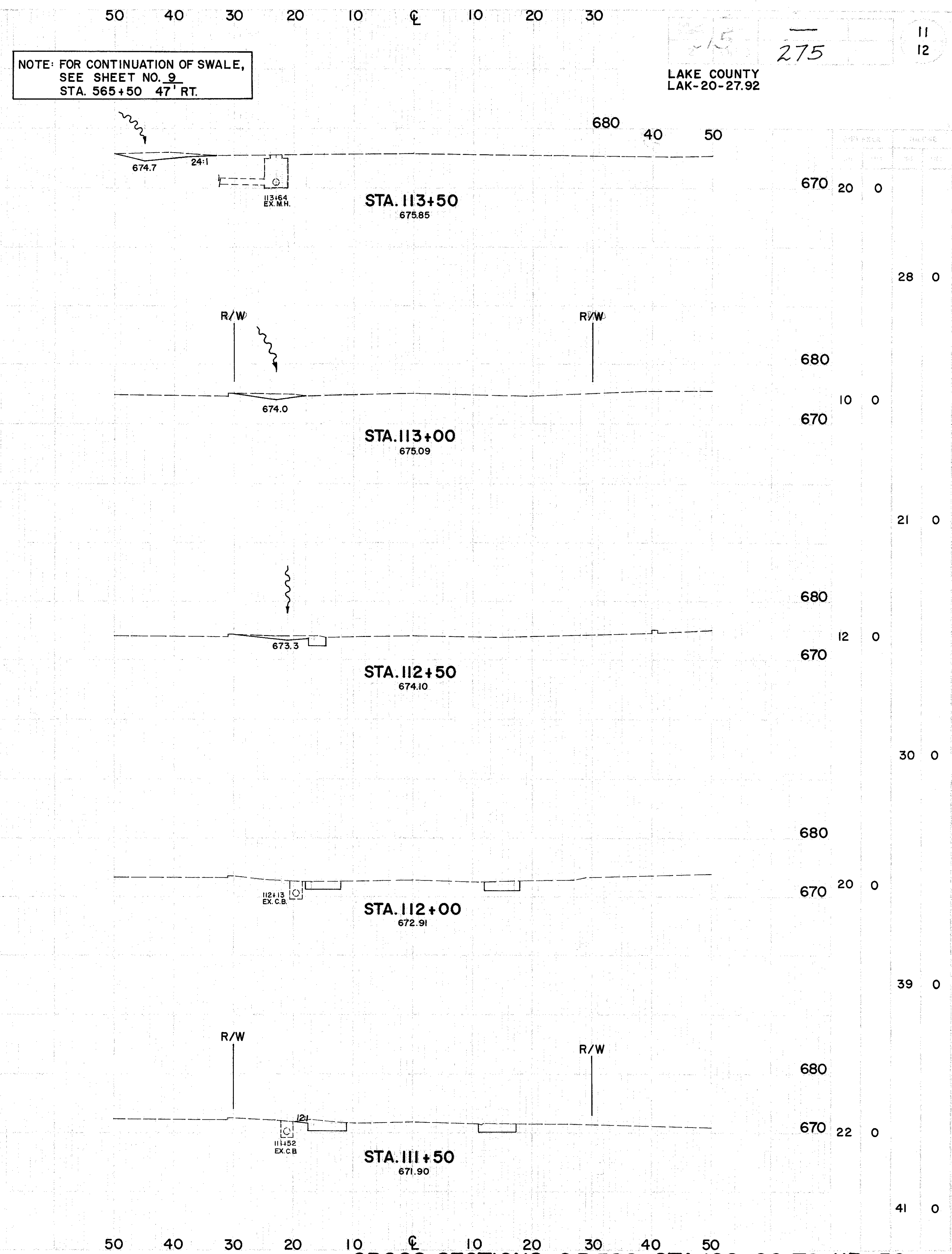
CROSS SECTIONS-S.R.528-STA.109+00 TO 113+50
