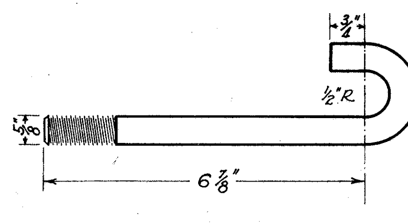
J BOLT
