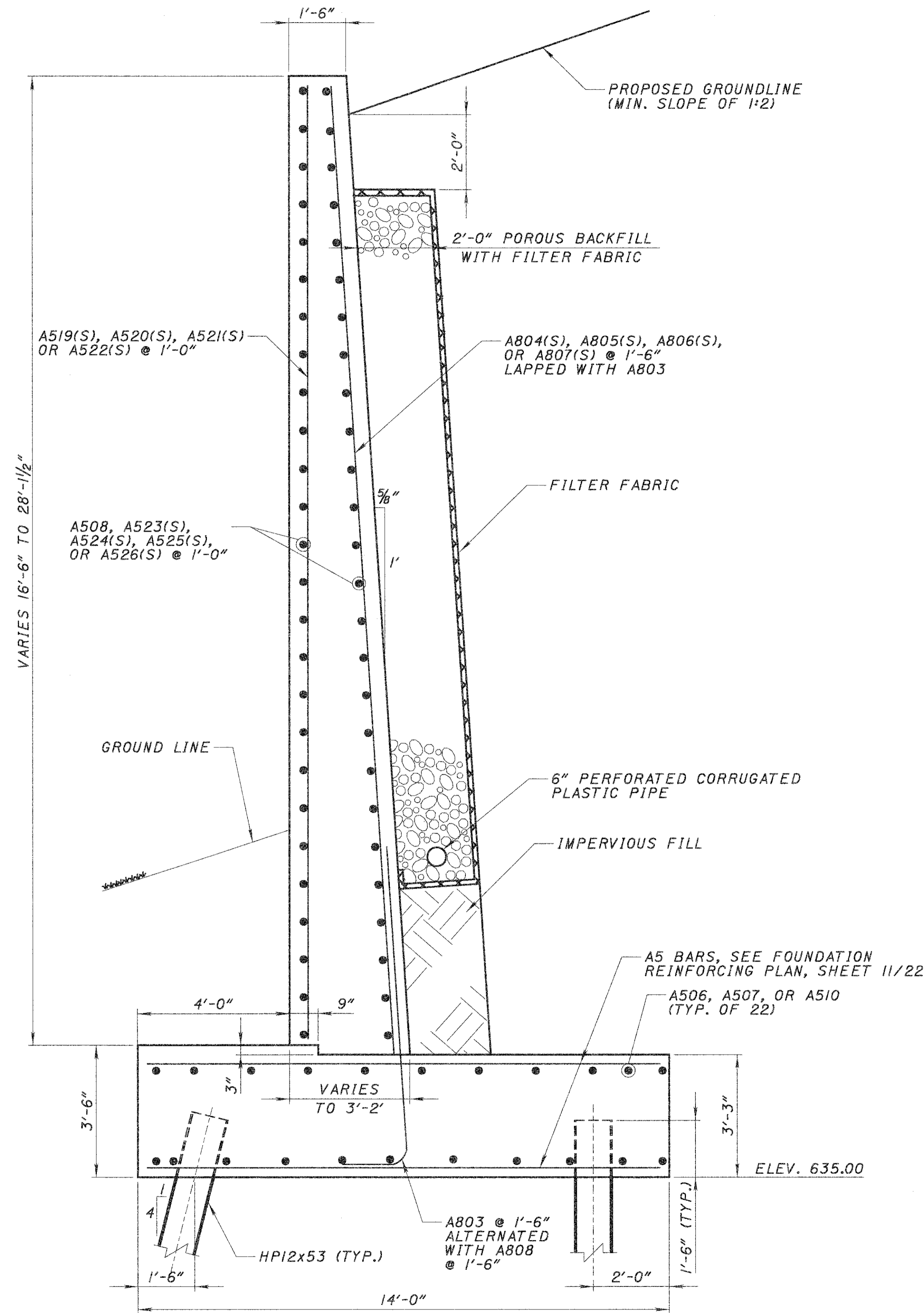
SECTION A-A
