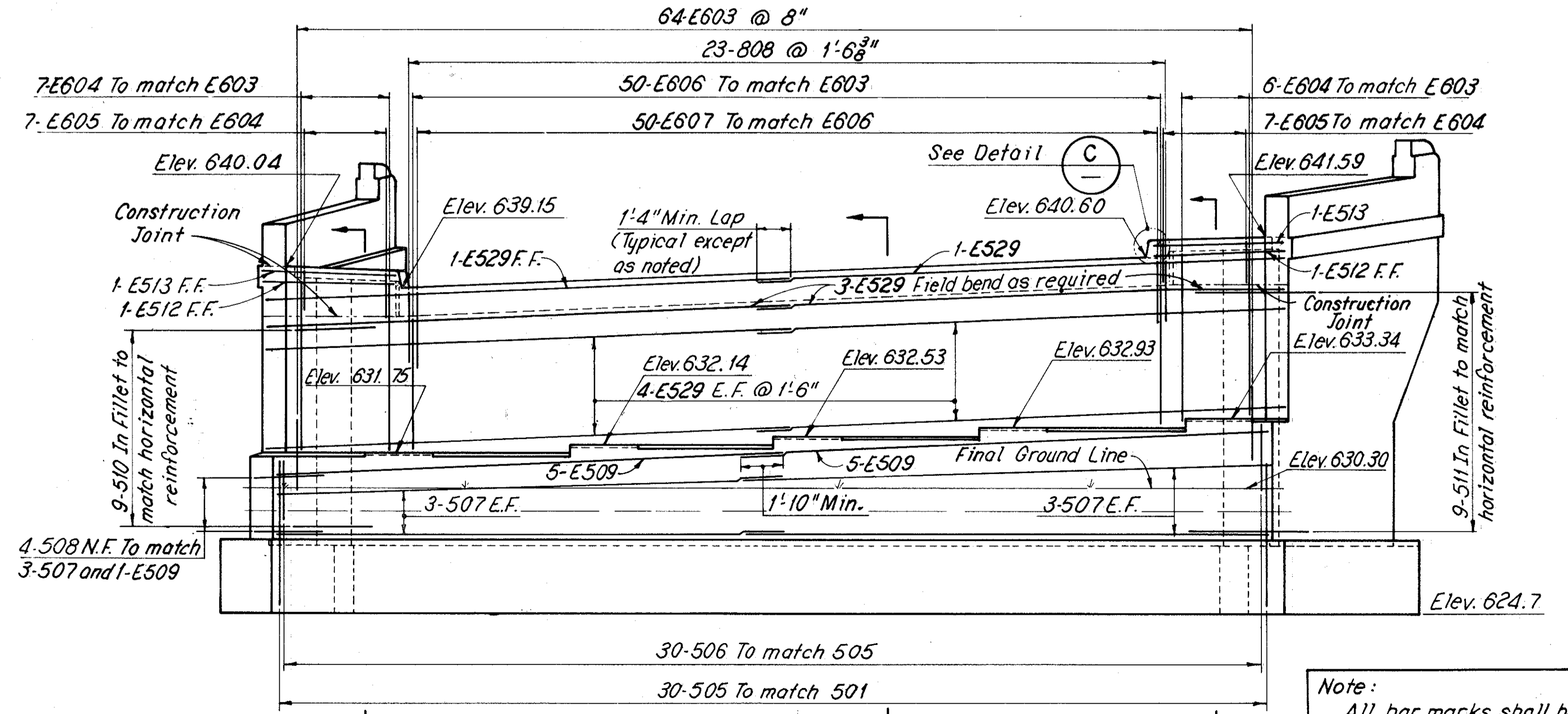
ELEVATION
