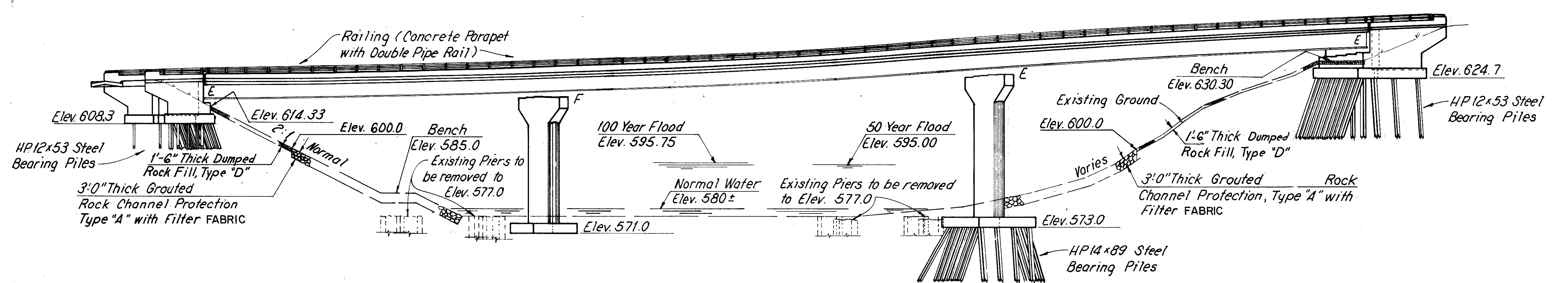
ELEVATION
