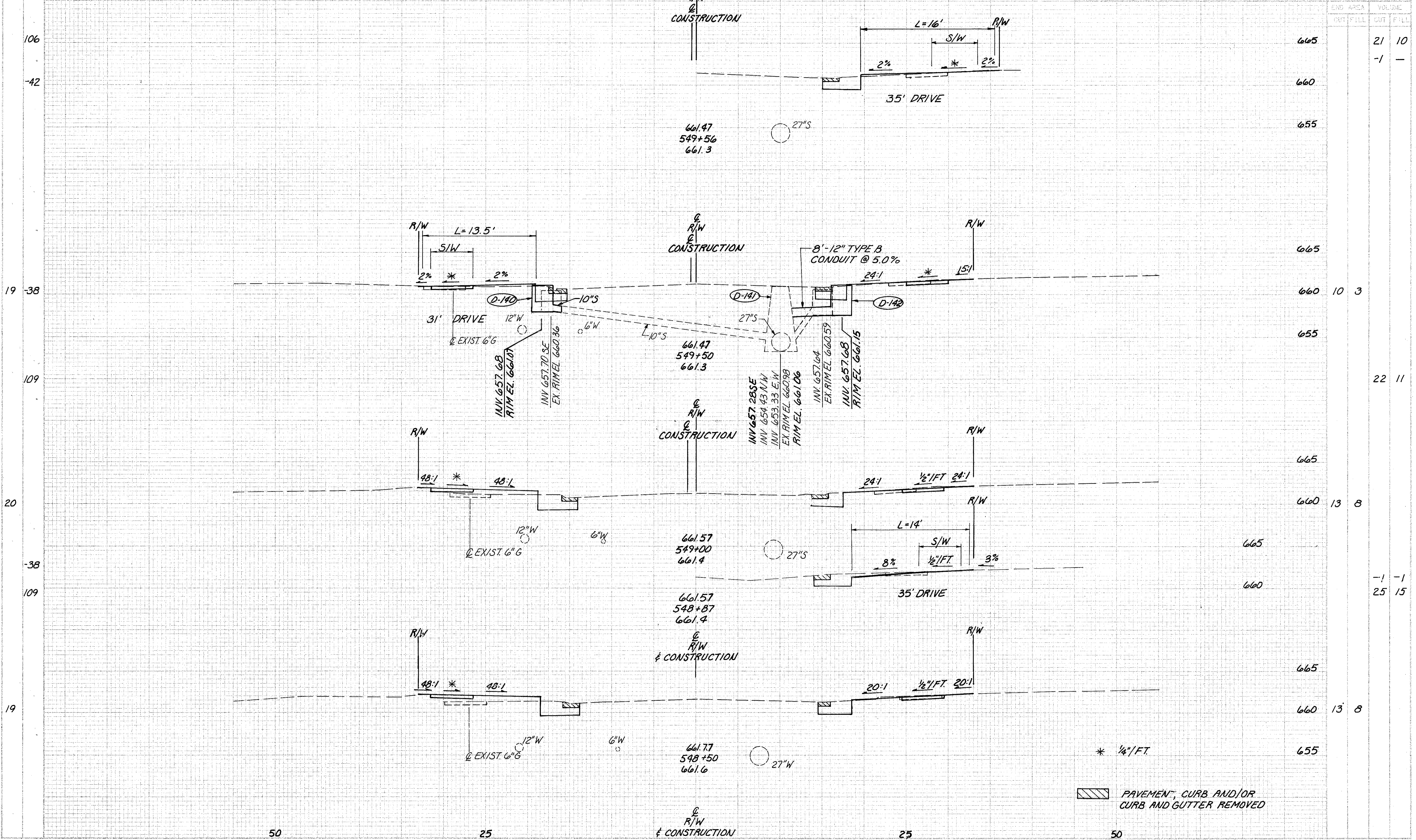
CROSS SECTIONS STA. 548+50 TO STA. 549+56
