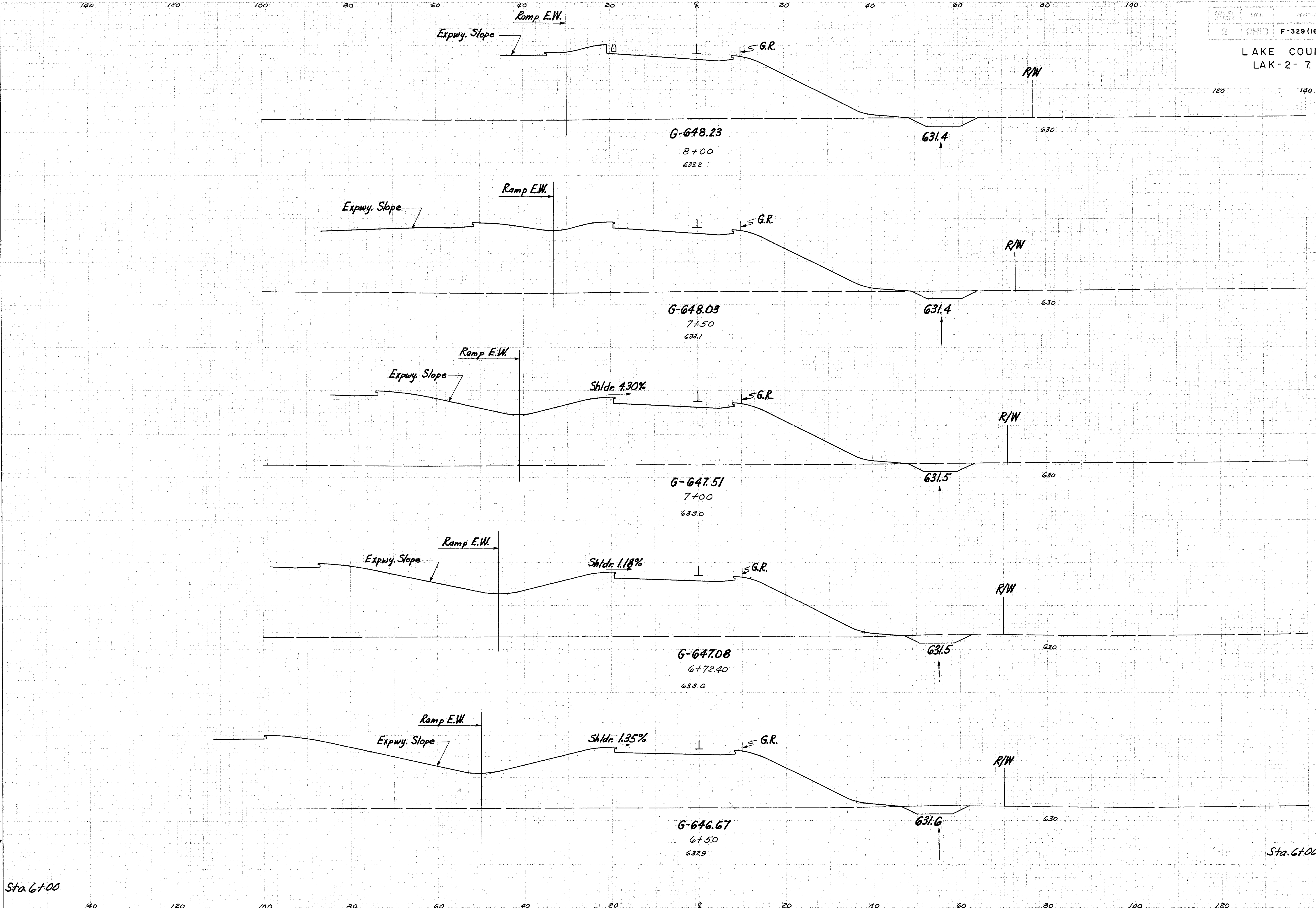
Ramp "T" Sta. 6+50 - 8+00
