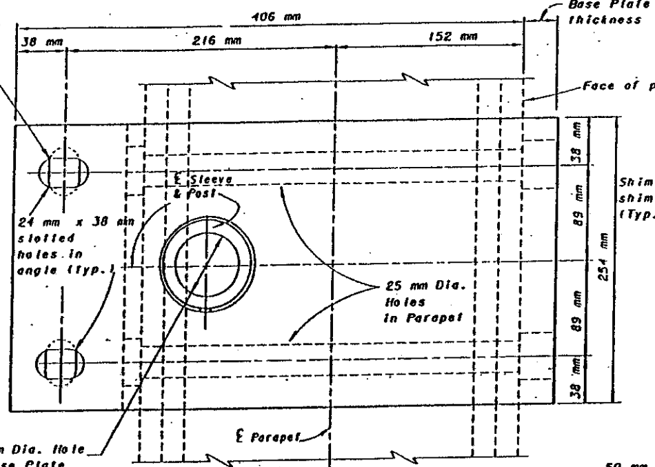
PLAN BP-4
