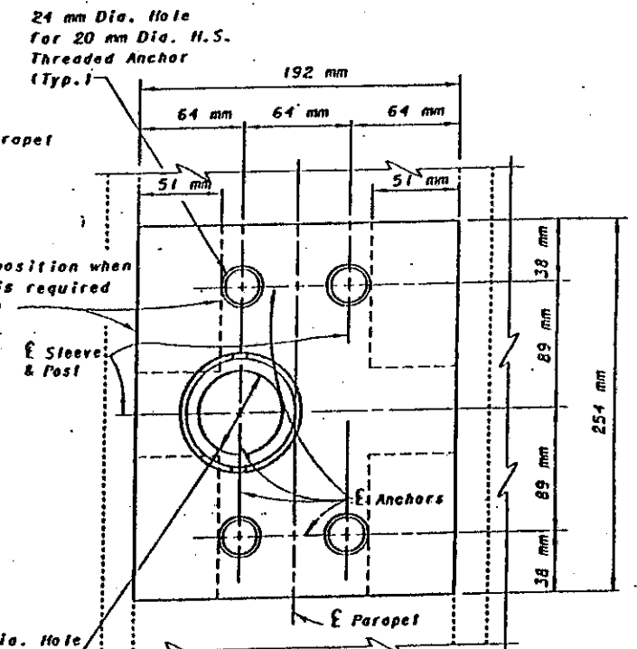
PLAN BP-5
