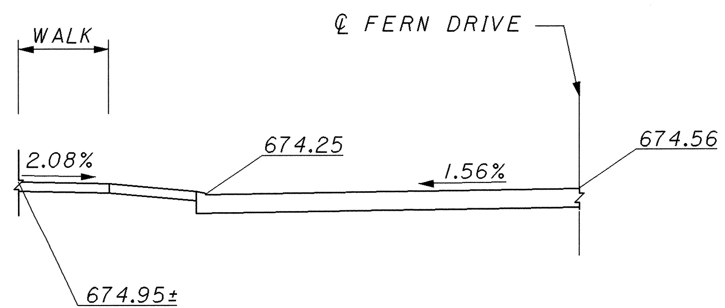
DETAIL A-A
