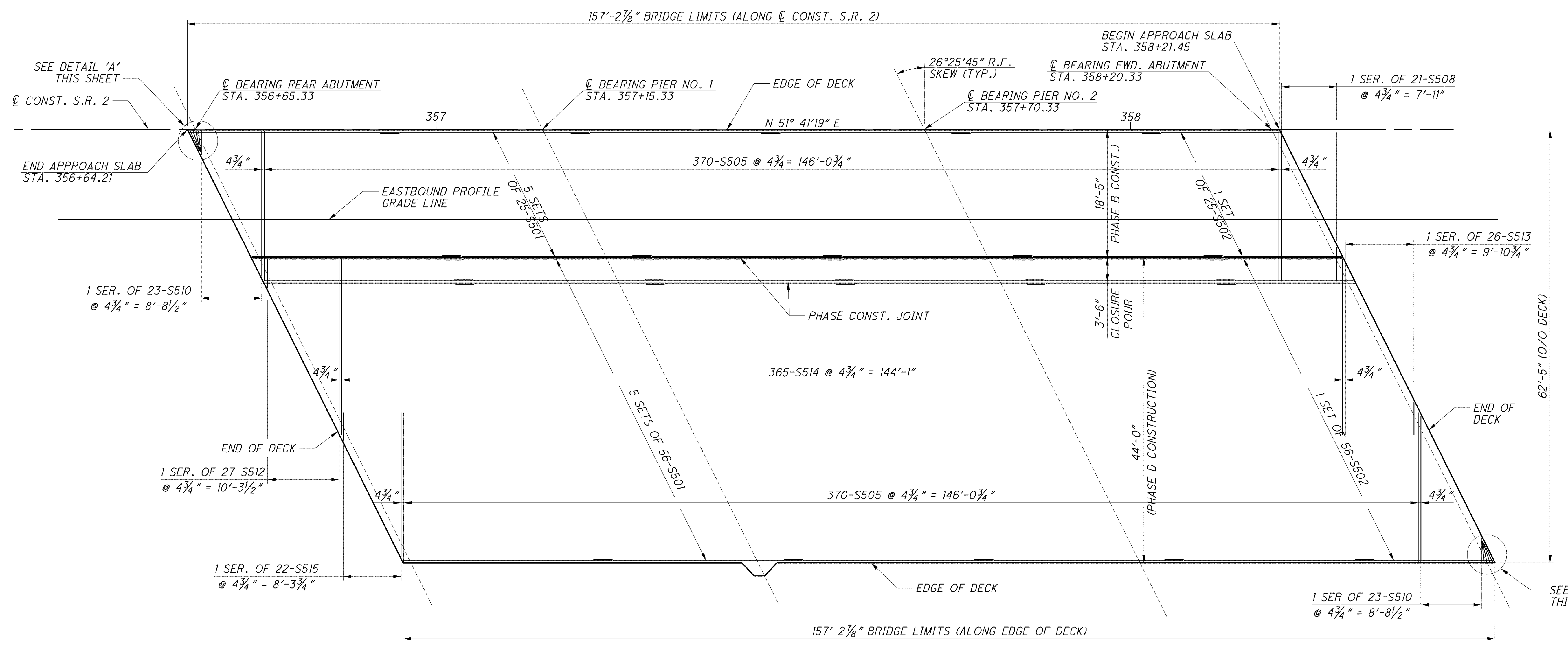
BOTTOM MAT
