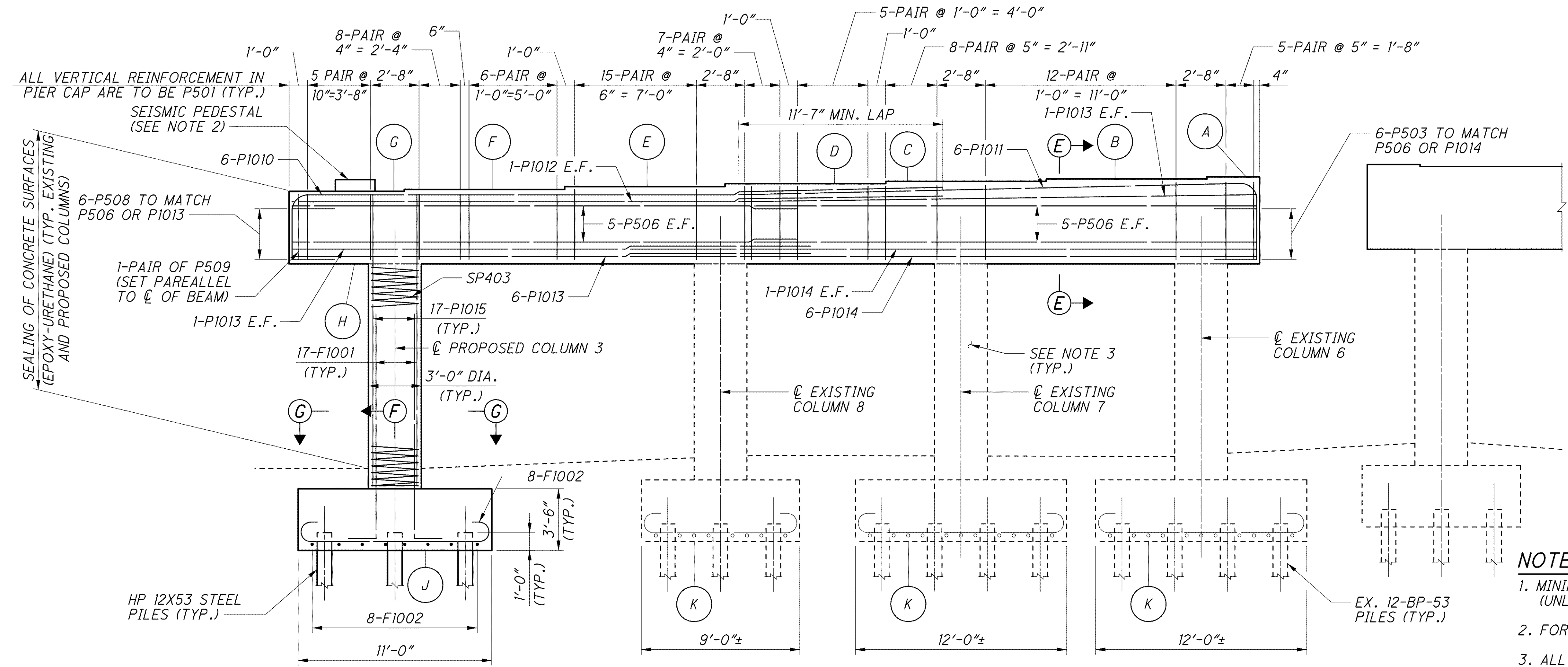
ELEVATION
