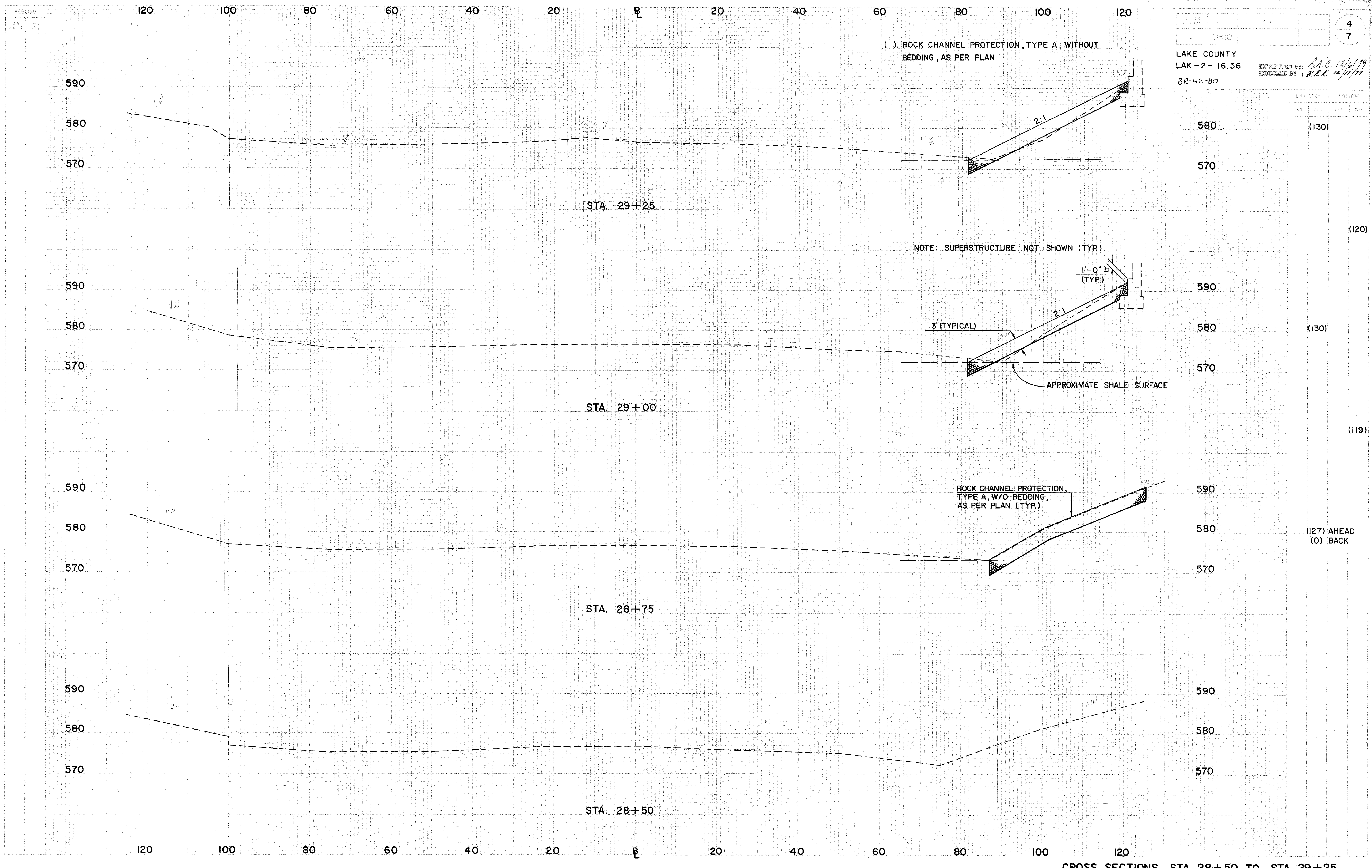
CROSS SECTIONS STA. 28+50 TO STA. 29+25
