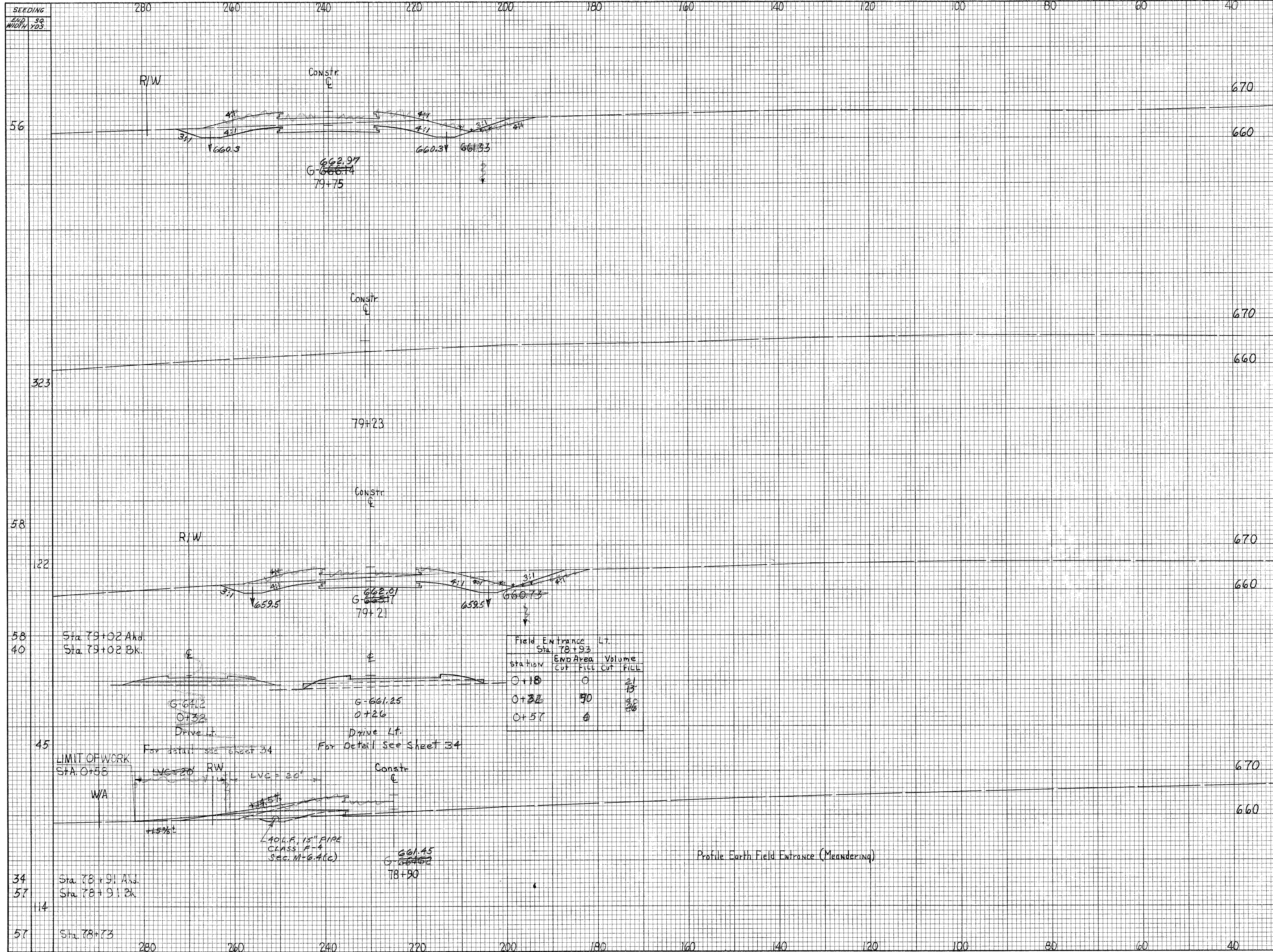
FRONTAGE ROAD "B" Sta. 78+90 to Sta. 79+72
