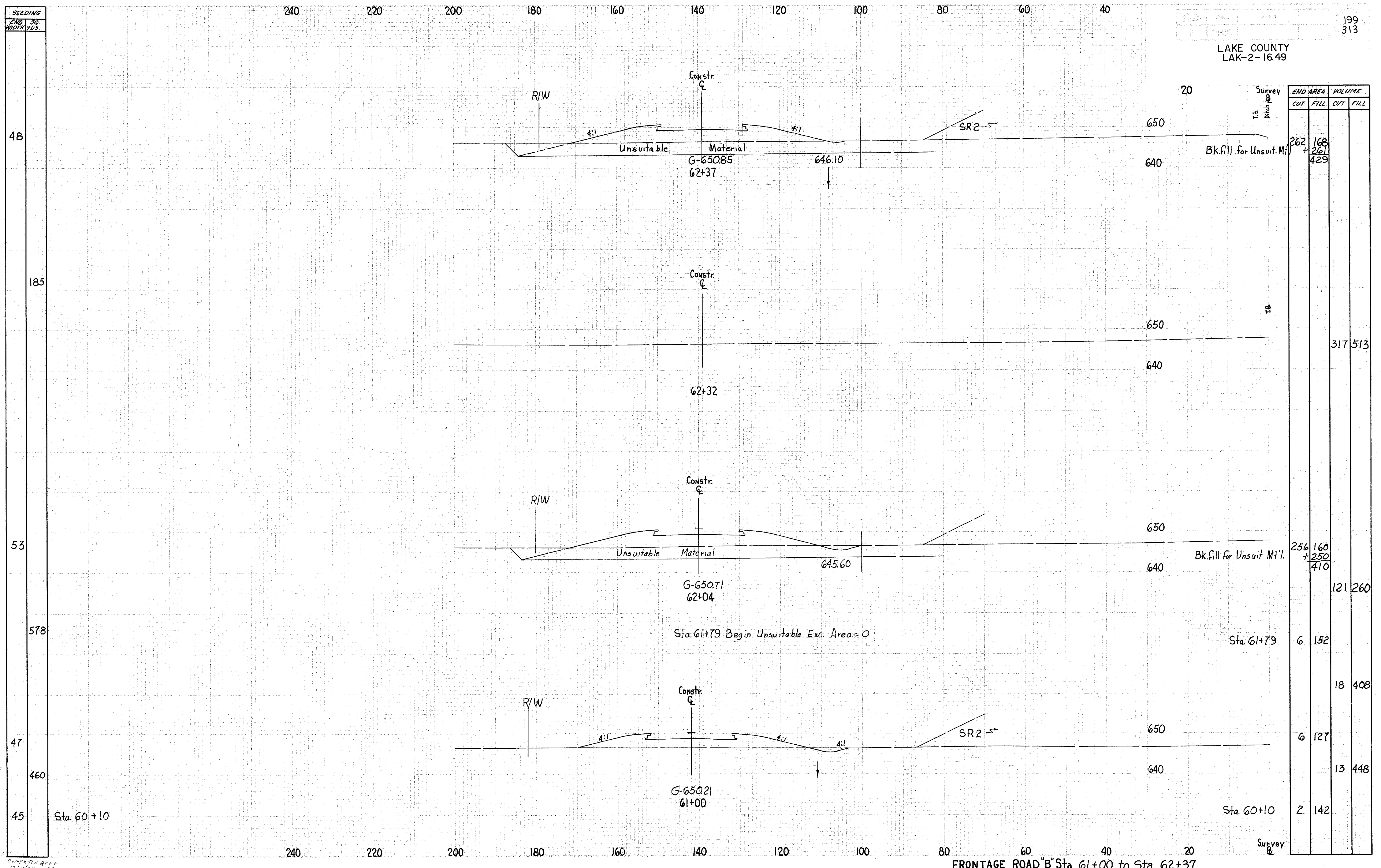
FRONTAGE ROAD "B" Sta. 61+00 to Sta. 62+37
