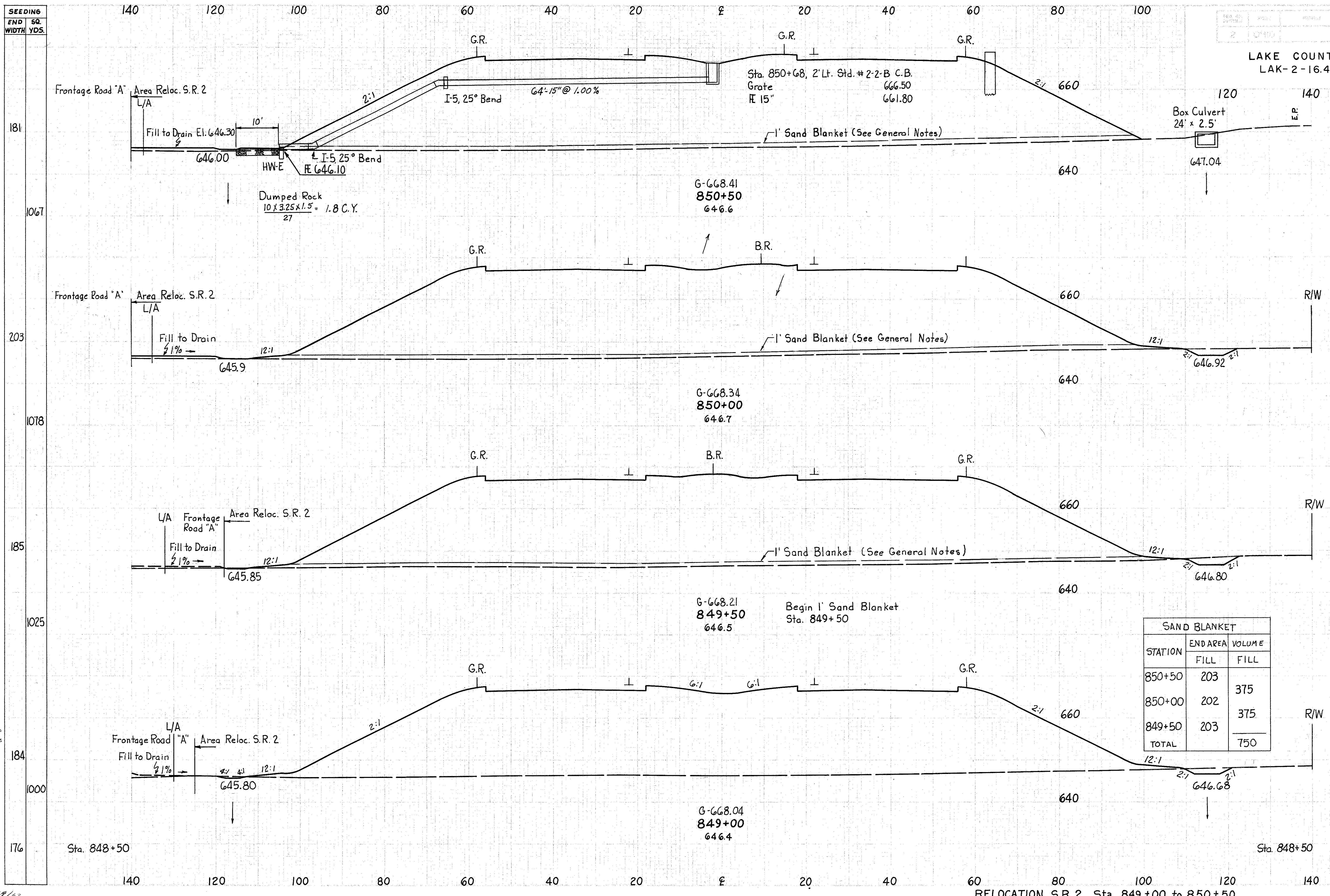
RELOCATION S.R. 2 Sta. 849+00 to 850+50
