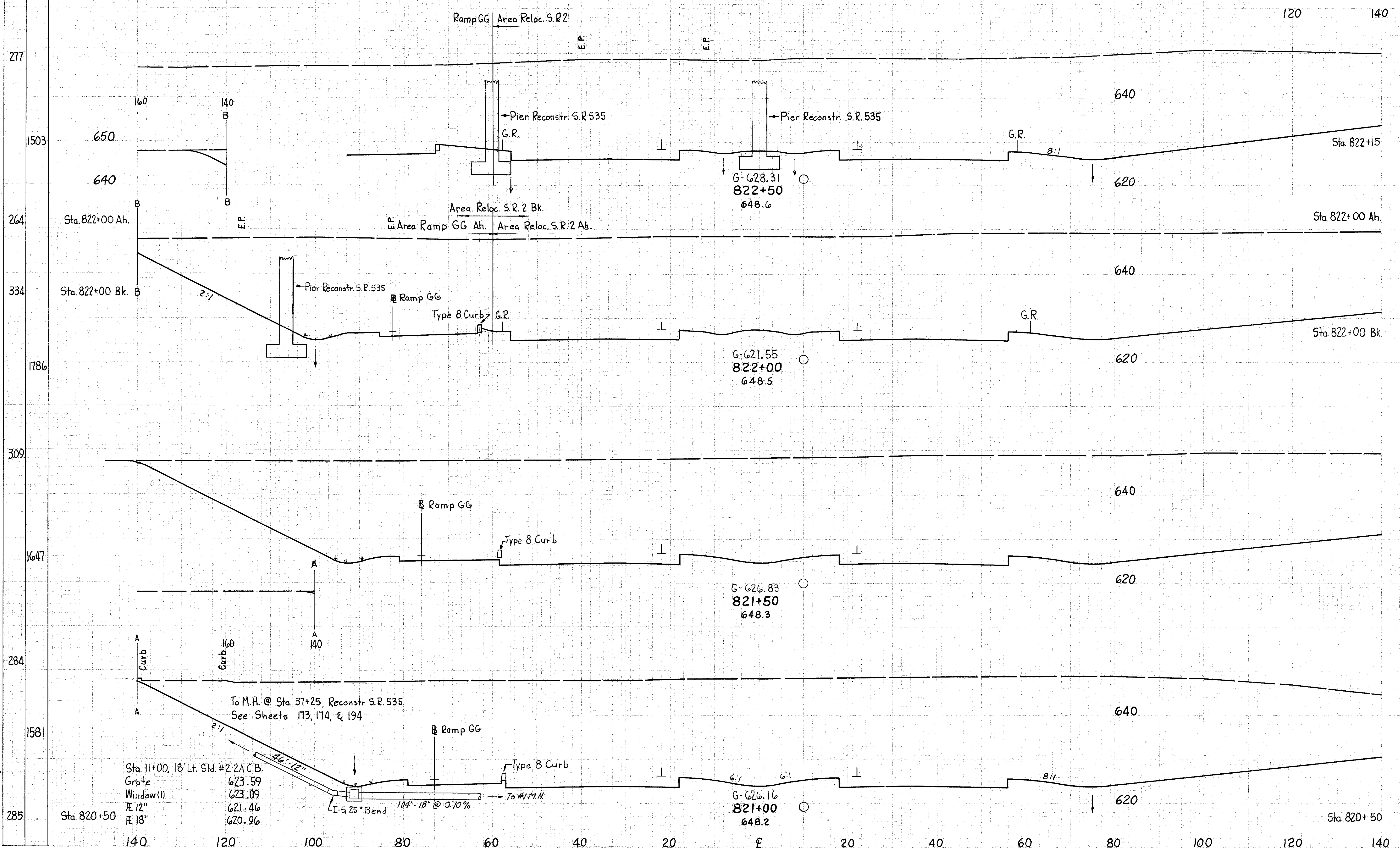
RELOCATION S.R. 2 Sta. 821+00 to 822+50
