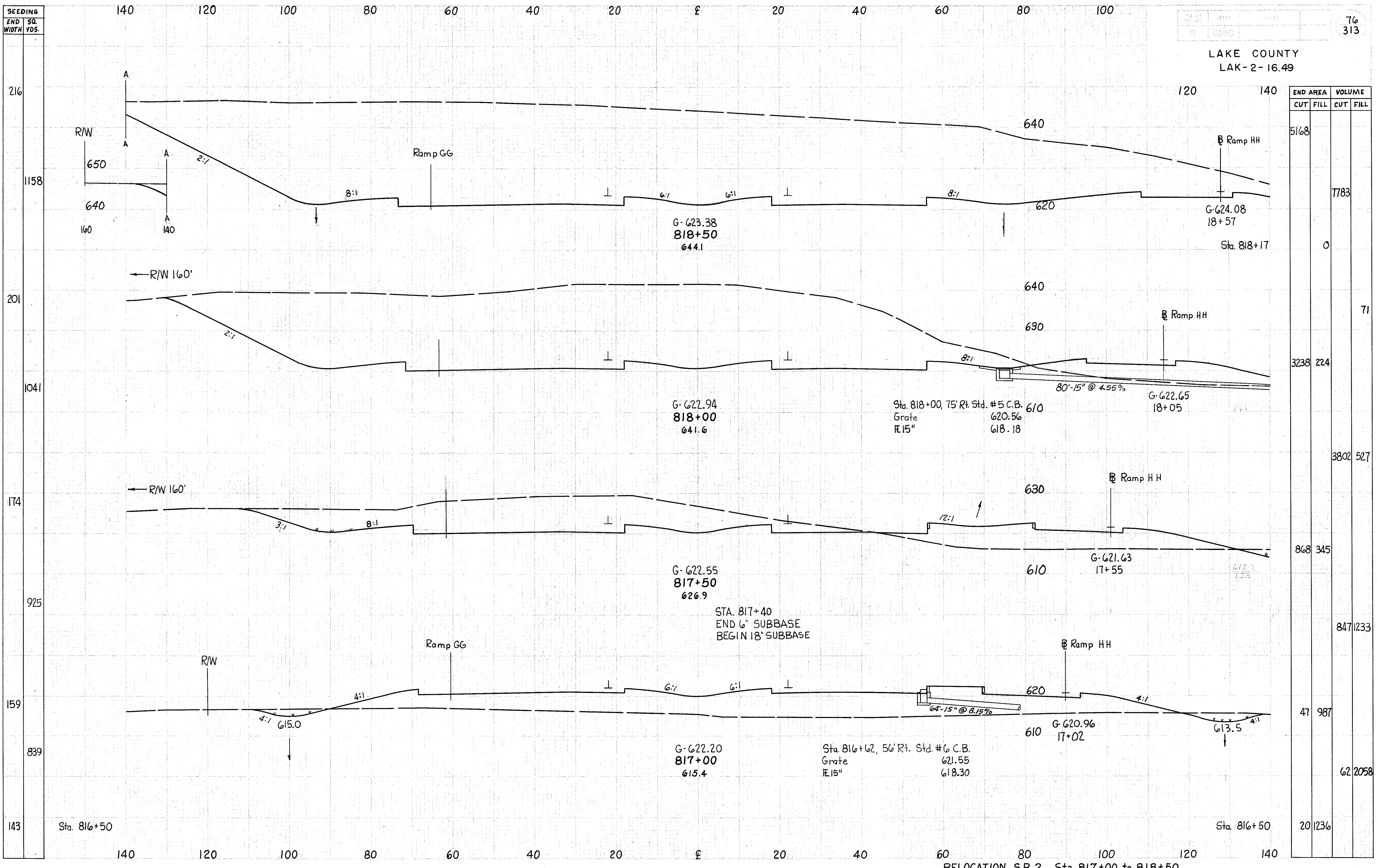
RELOCATION S.R.2 Sta. 817+00 to 818+50
