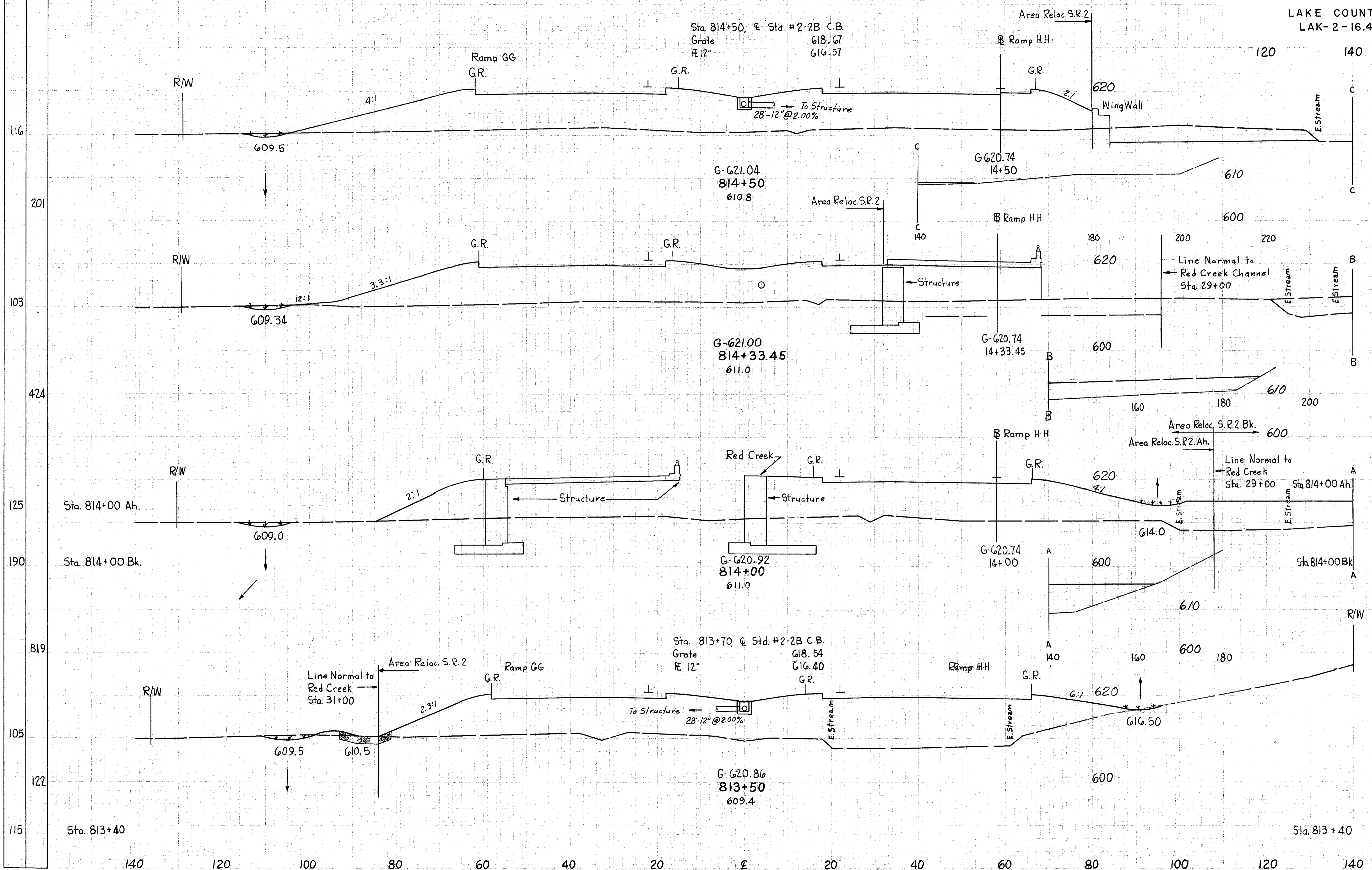
RELOCATION S.R. 2 Sta. 813+50 to 814+50
