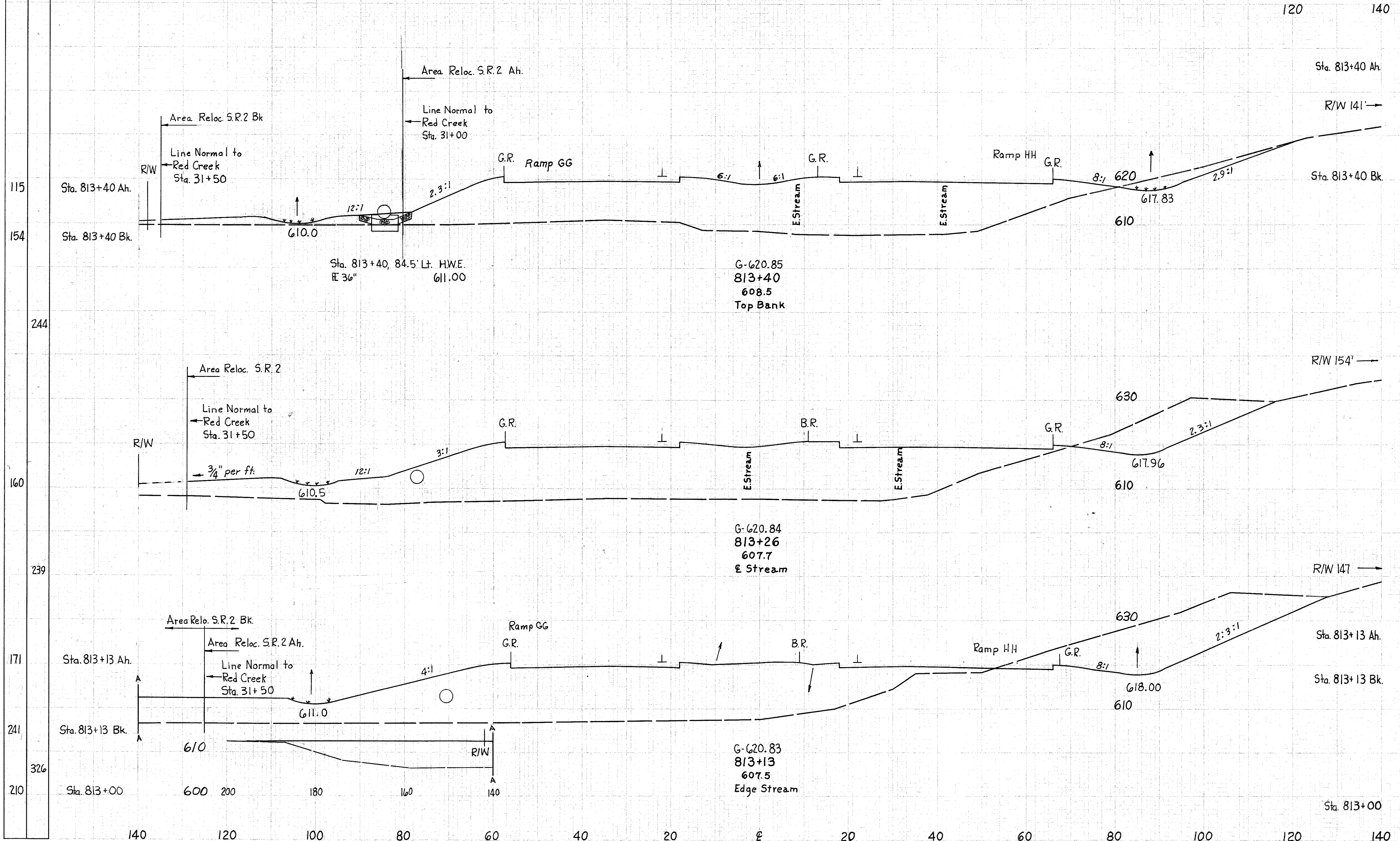
RELOCATION S.R.2 Sta. 813+13 to 813+40
