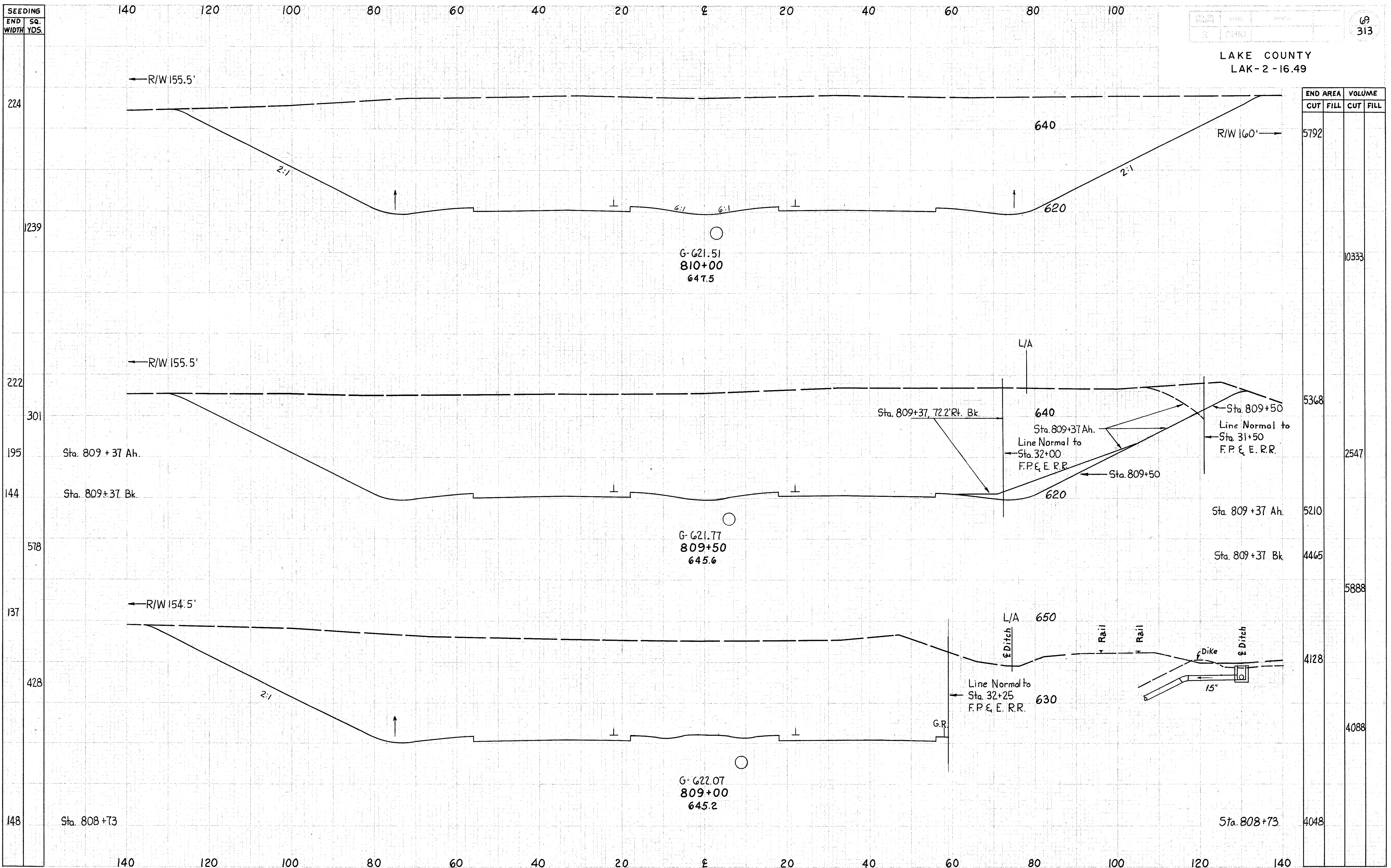
RELOCATION S.R. 2 Sta. 809+00 to 810+00
