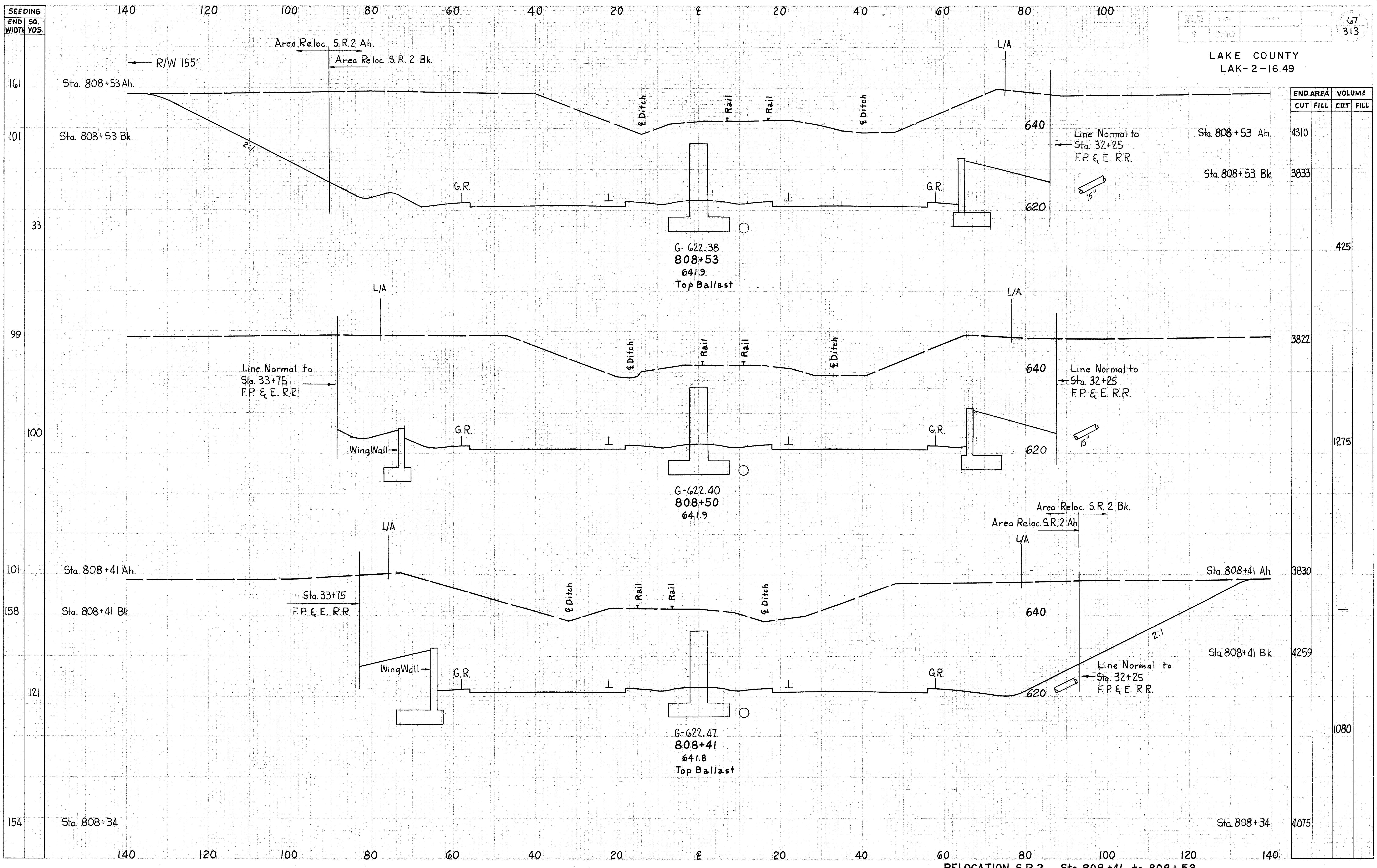
RELOCATION S.R. 2 Sta. 808+41 to 808+53
