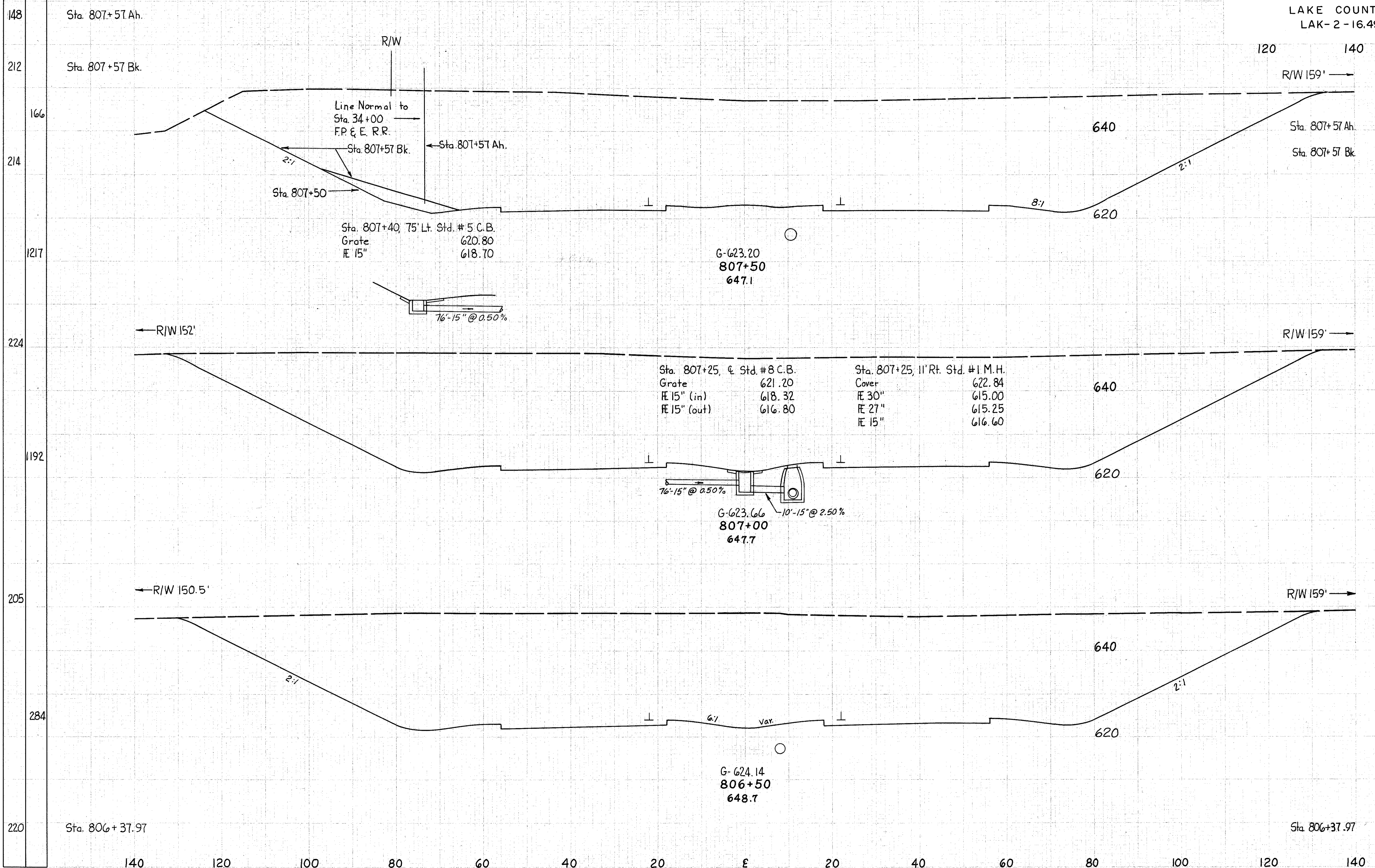
RELOCATION S.R.2 Sta. 806+50 to 807+50
