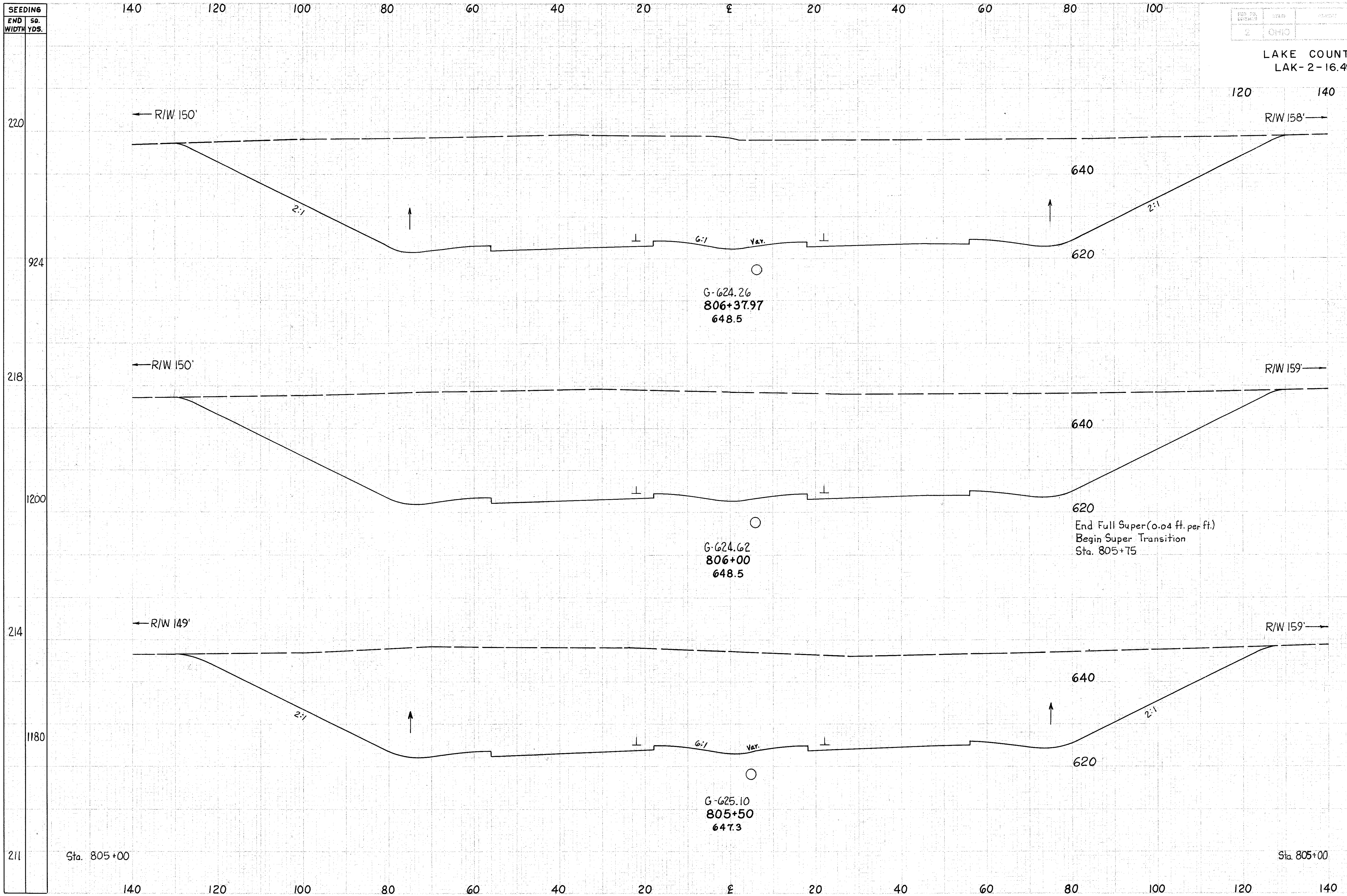
RELOCATION S.R. 2 Sta. 805+50 to 806+37.97.
