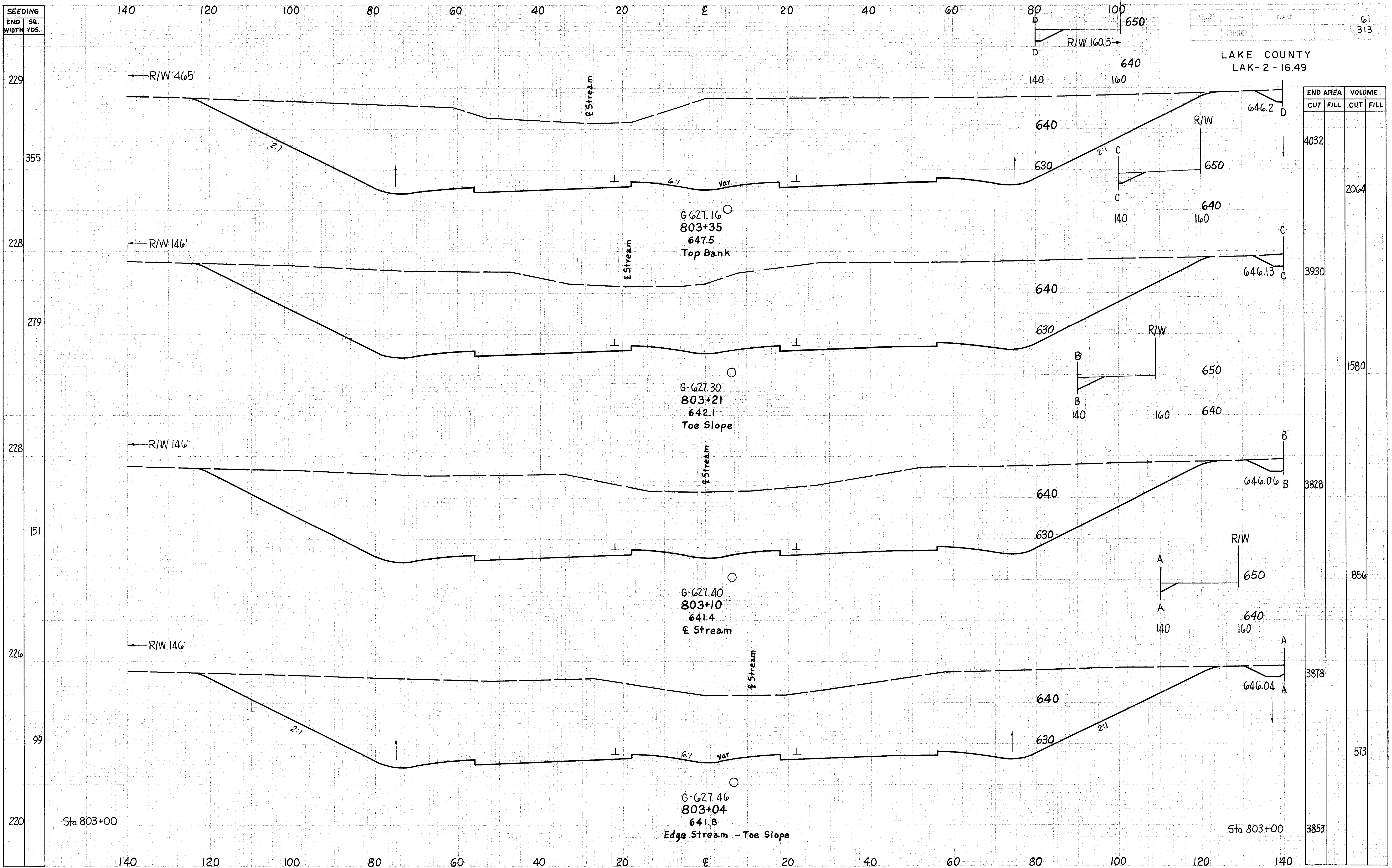
RELOCATION S.R.2 Sta. 803+04 to 803+35
