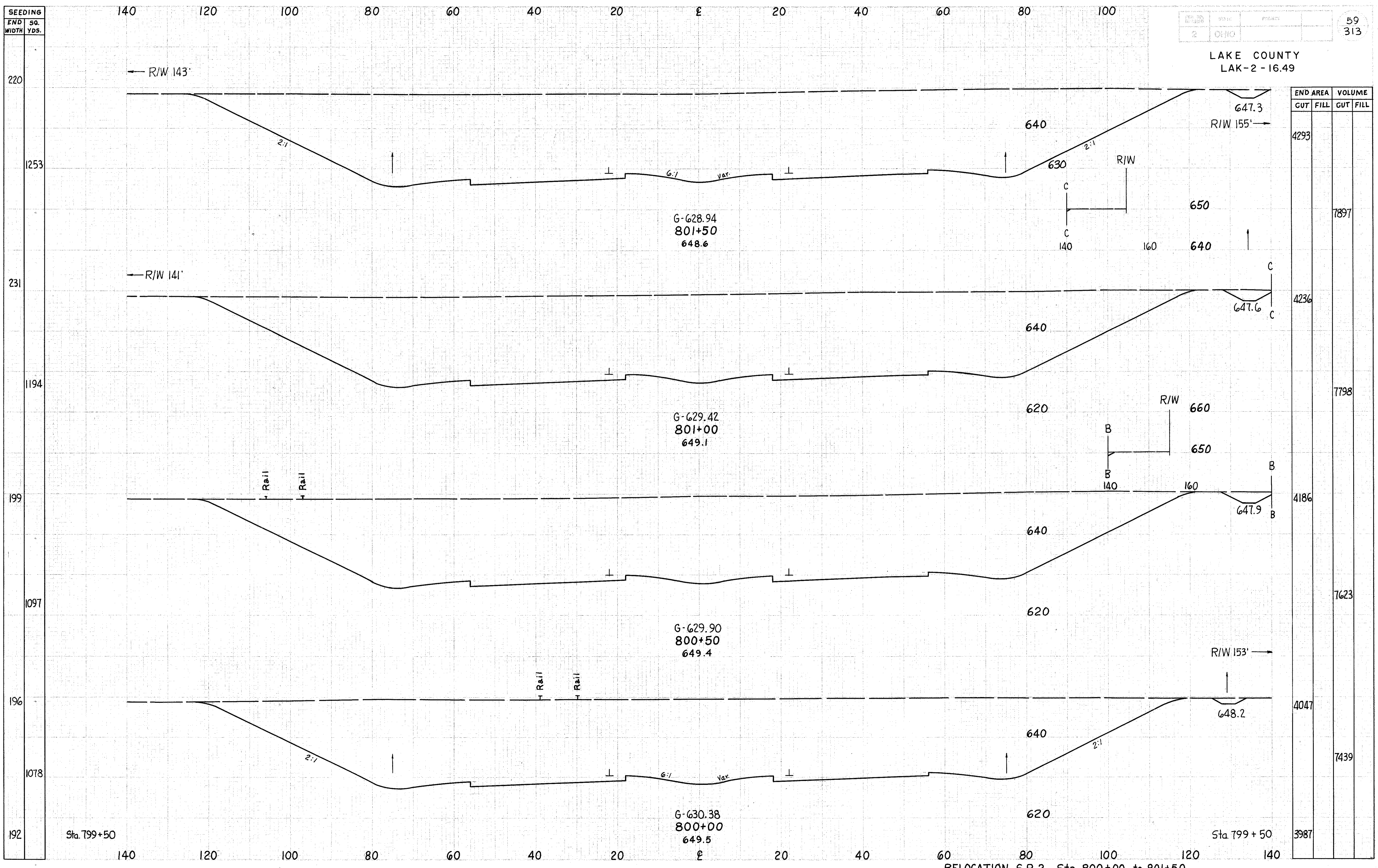
RELOCATION S.R.2 Sta. 800+00 to 801+50
