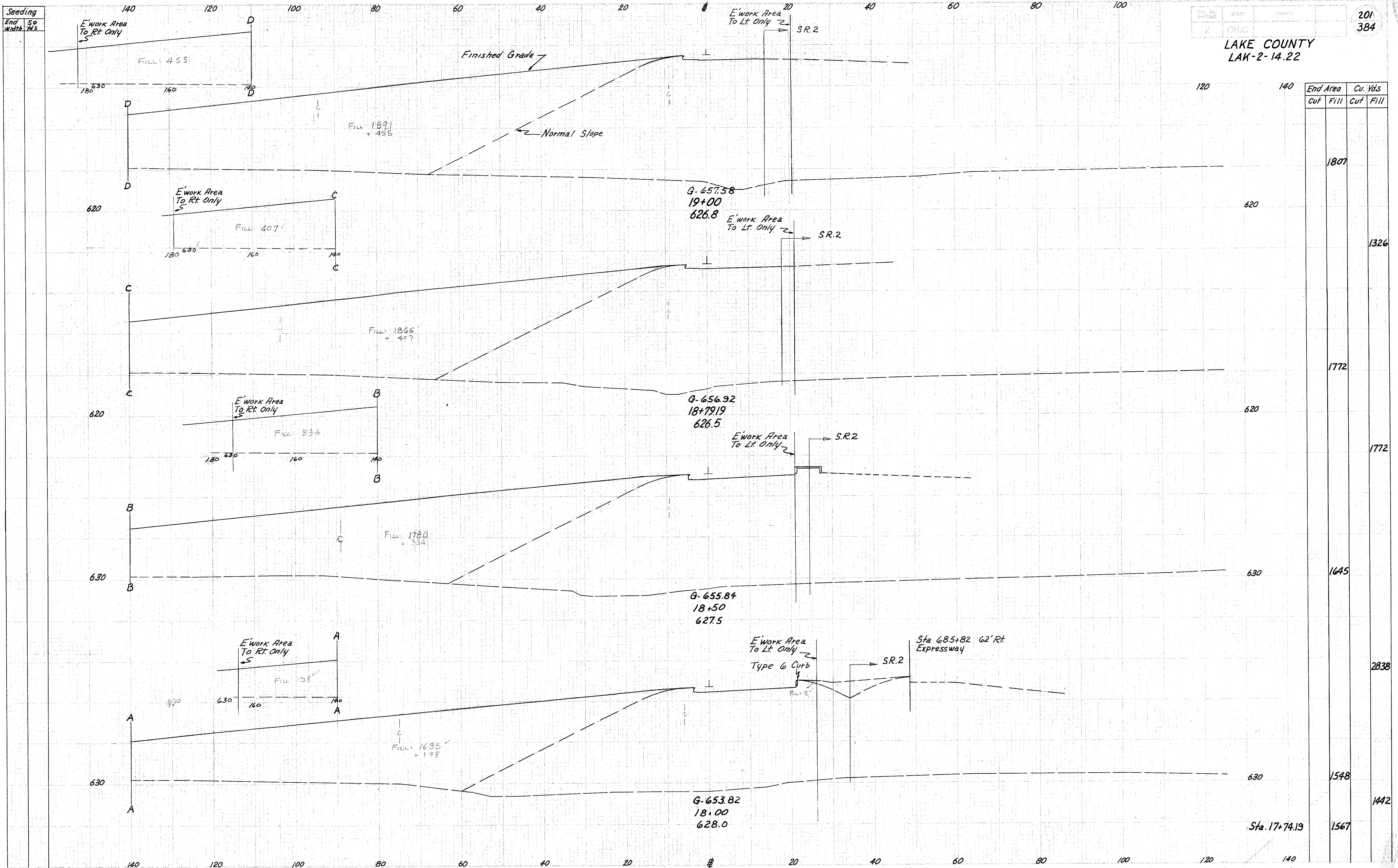
Ramp "EE" Sta. 18+00 to Sta. 19+00
