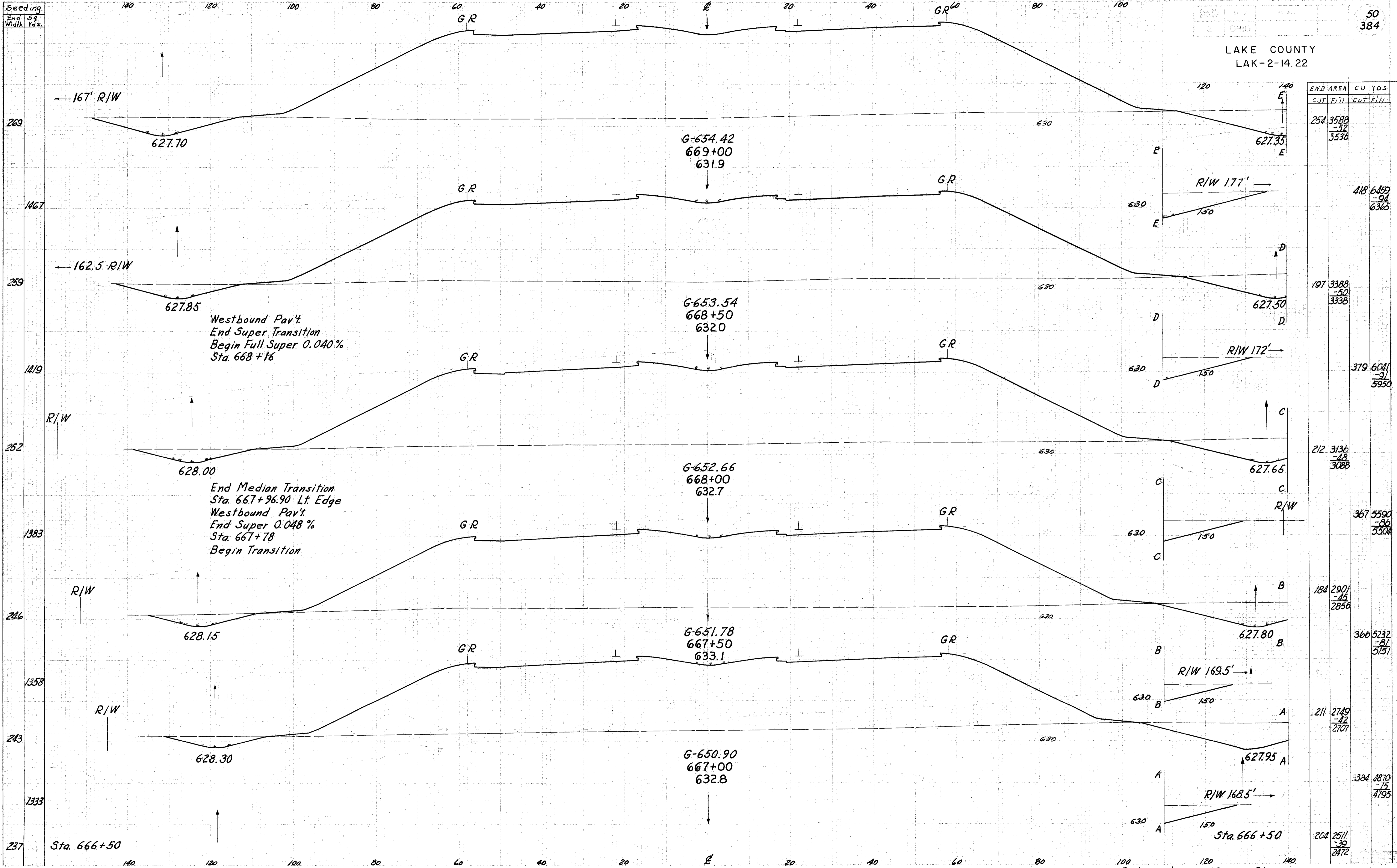
Relocation SR.2 Sta. 667+00 to 669+00
