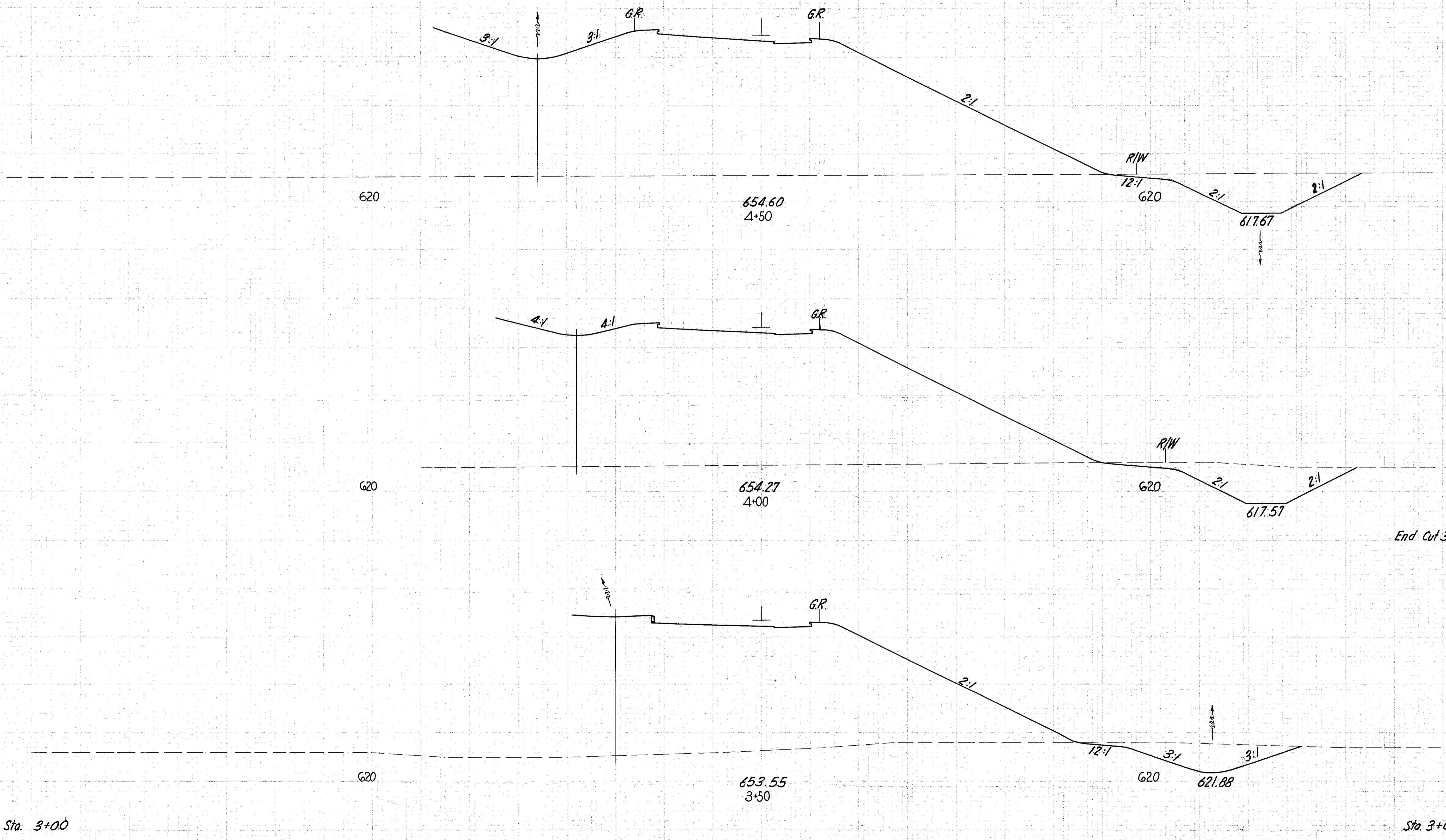
Ramp H Sta. 3+50 to 4+50
