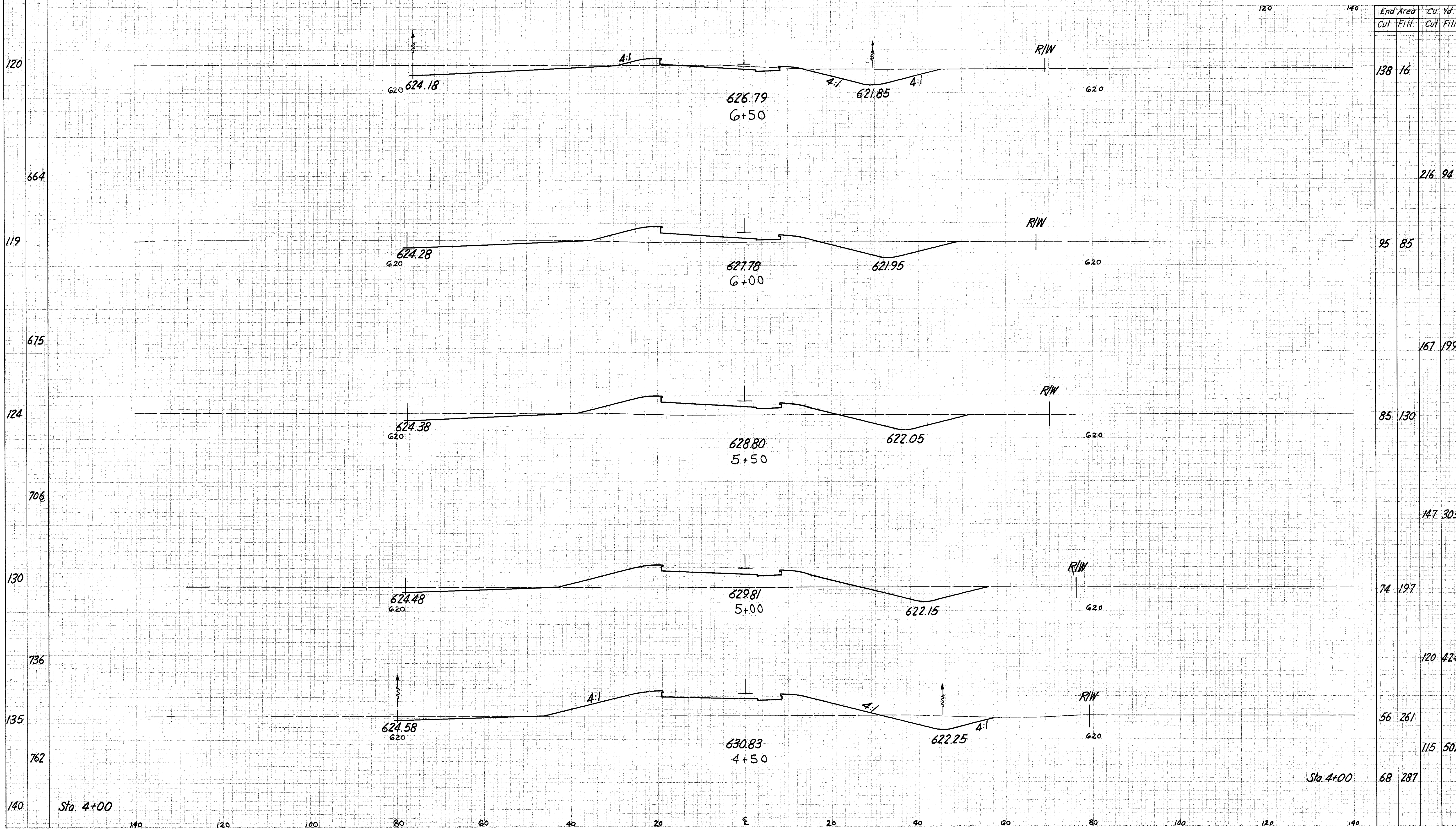
Ramp 'C' Sta. 4+50 to G+50
