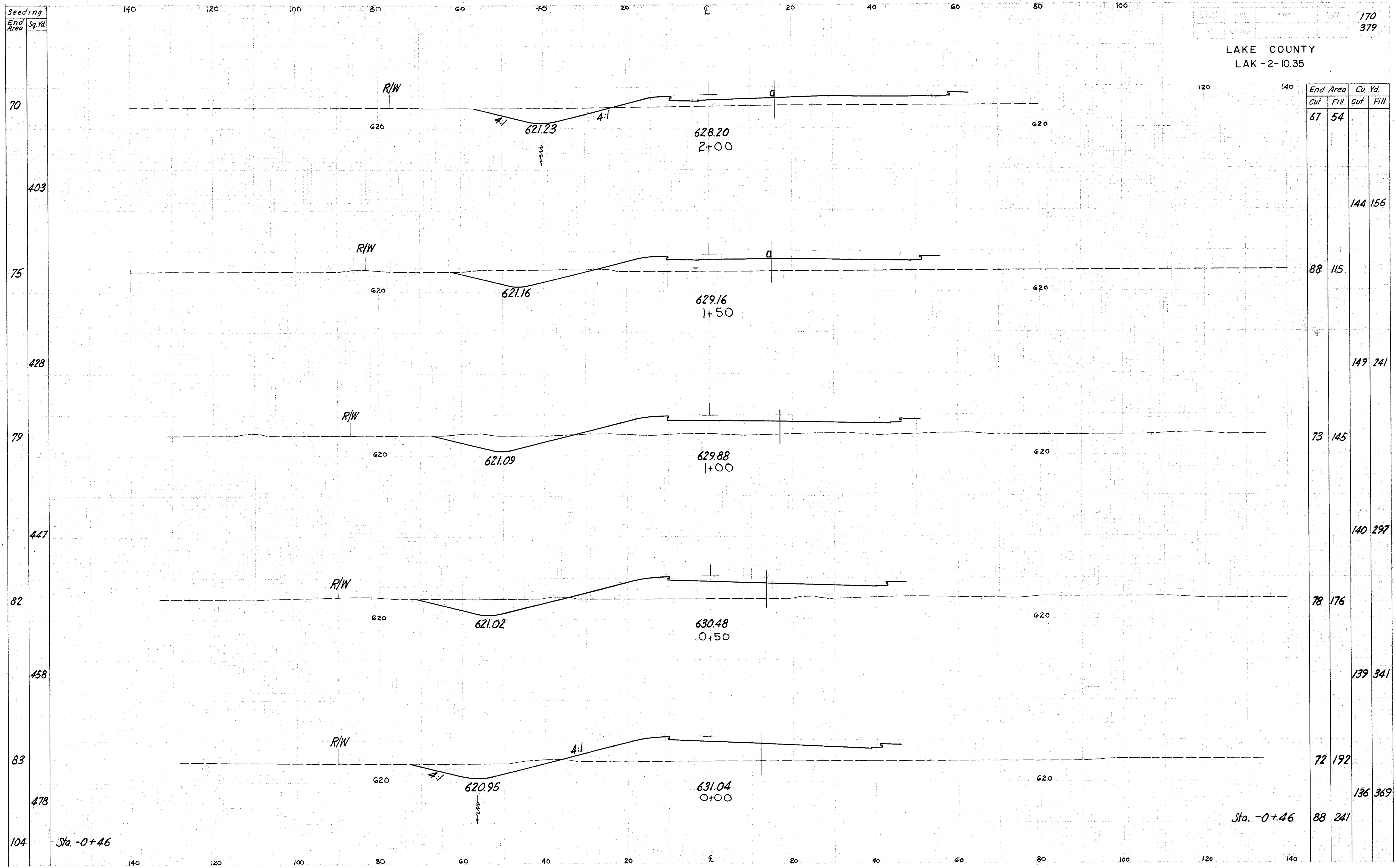
Ramp 'A' STA. 0+00 to 2+00
