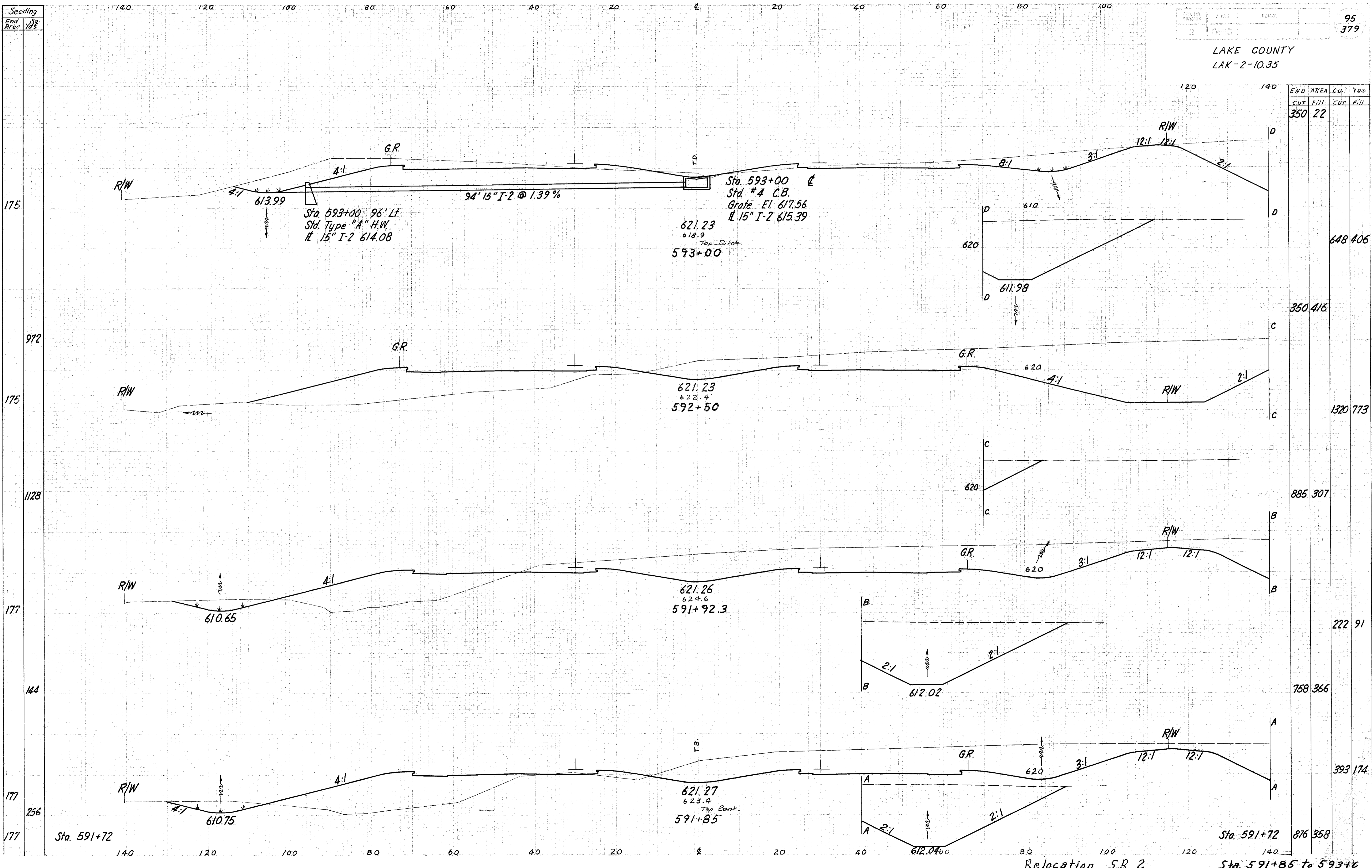
Relocation S.R 2 Sta. 591+85 to 593+72
