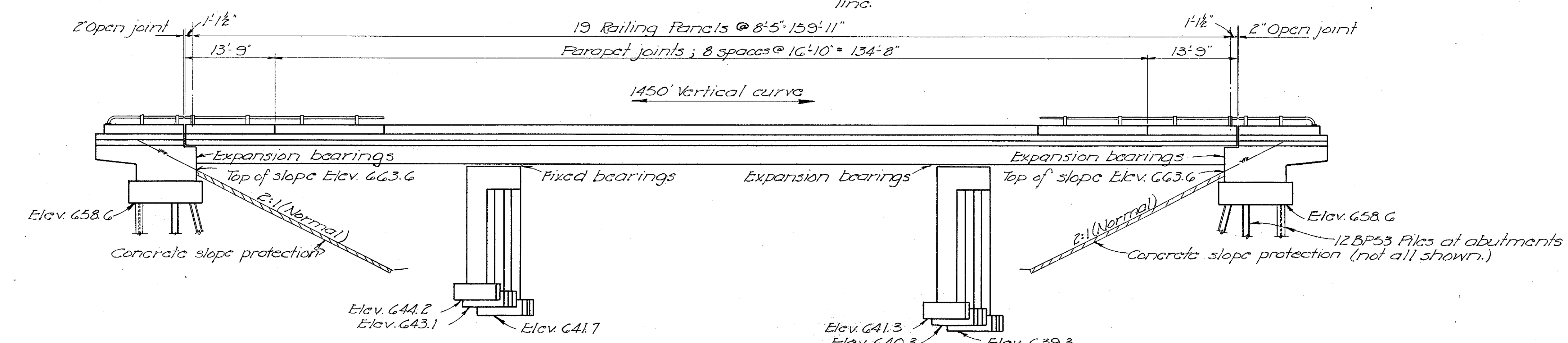
ELEVATION
