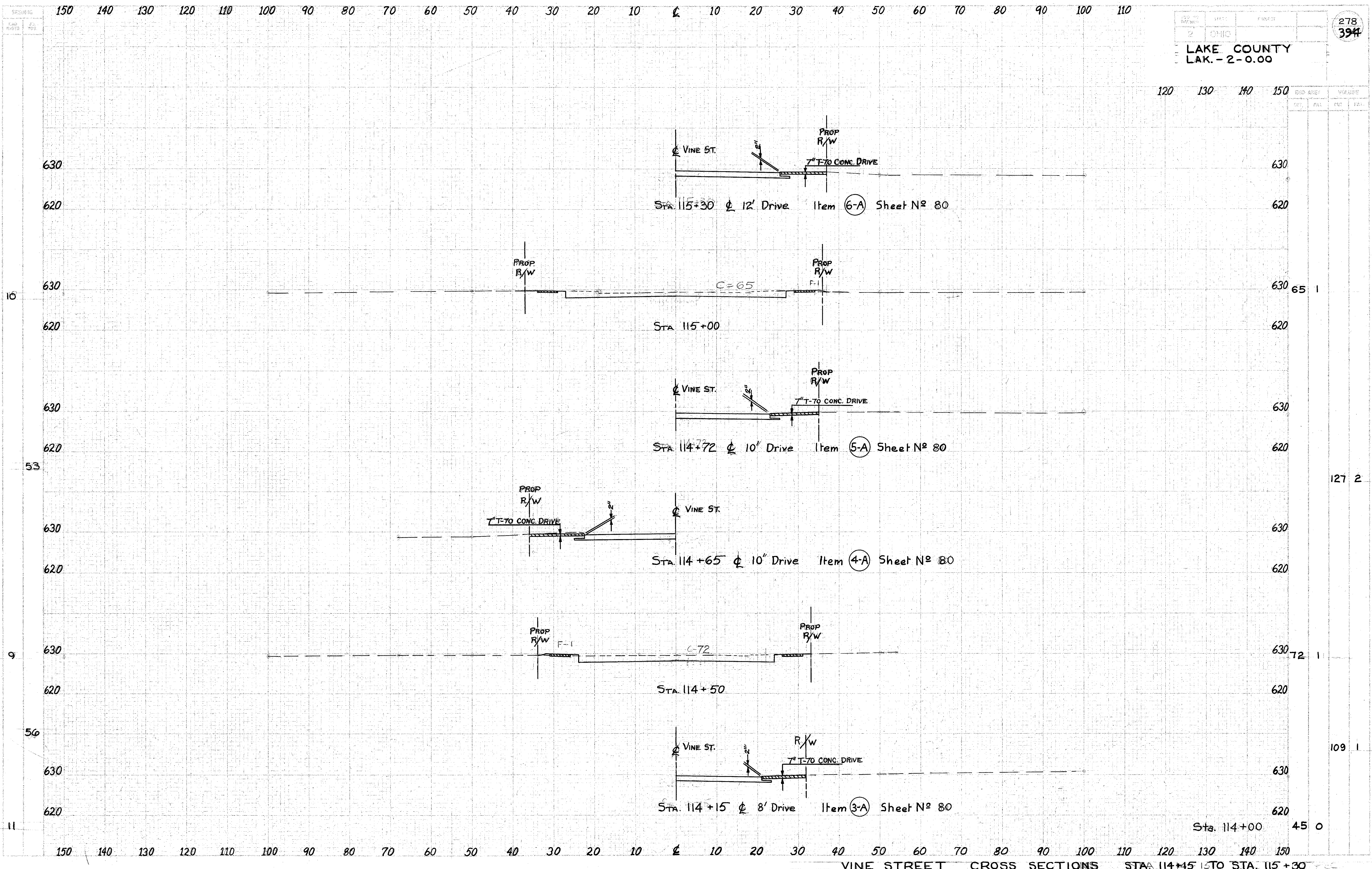
VINE STREET CROSS SECTIONS STA. 114+00 TO STA. 115+30
